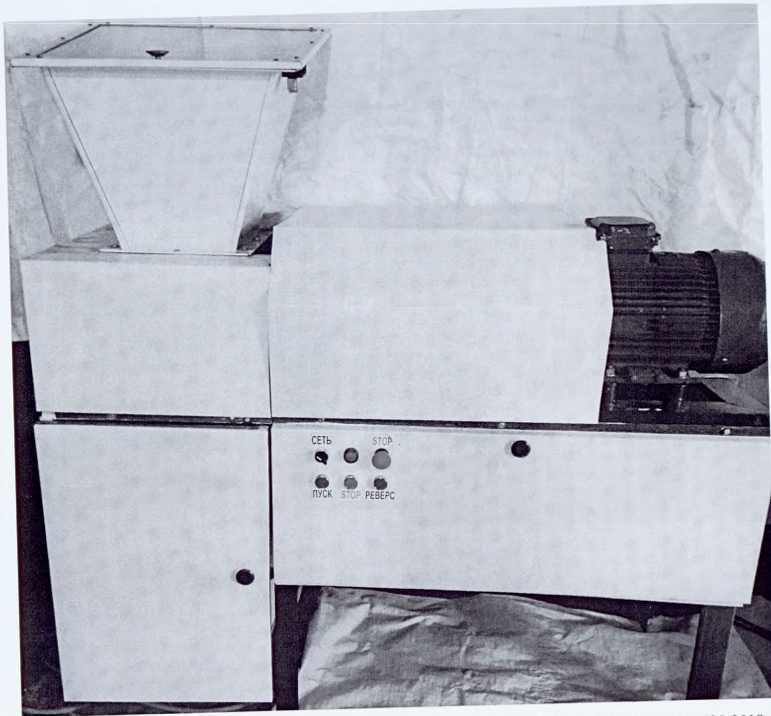
ООО ЦРМИ info@cirmi.ru www.goszdravnadzor.ru заражения медицинских отходов микроволновая «Бионар» по ТУ 32.50.50-001-20851585-2018: Общий вид устройства измельчения отходов
