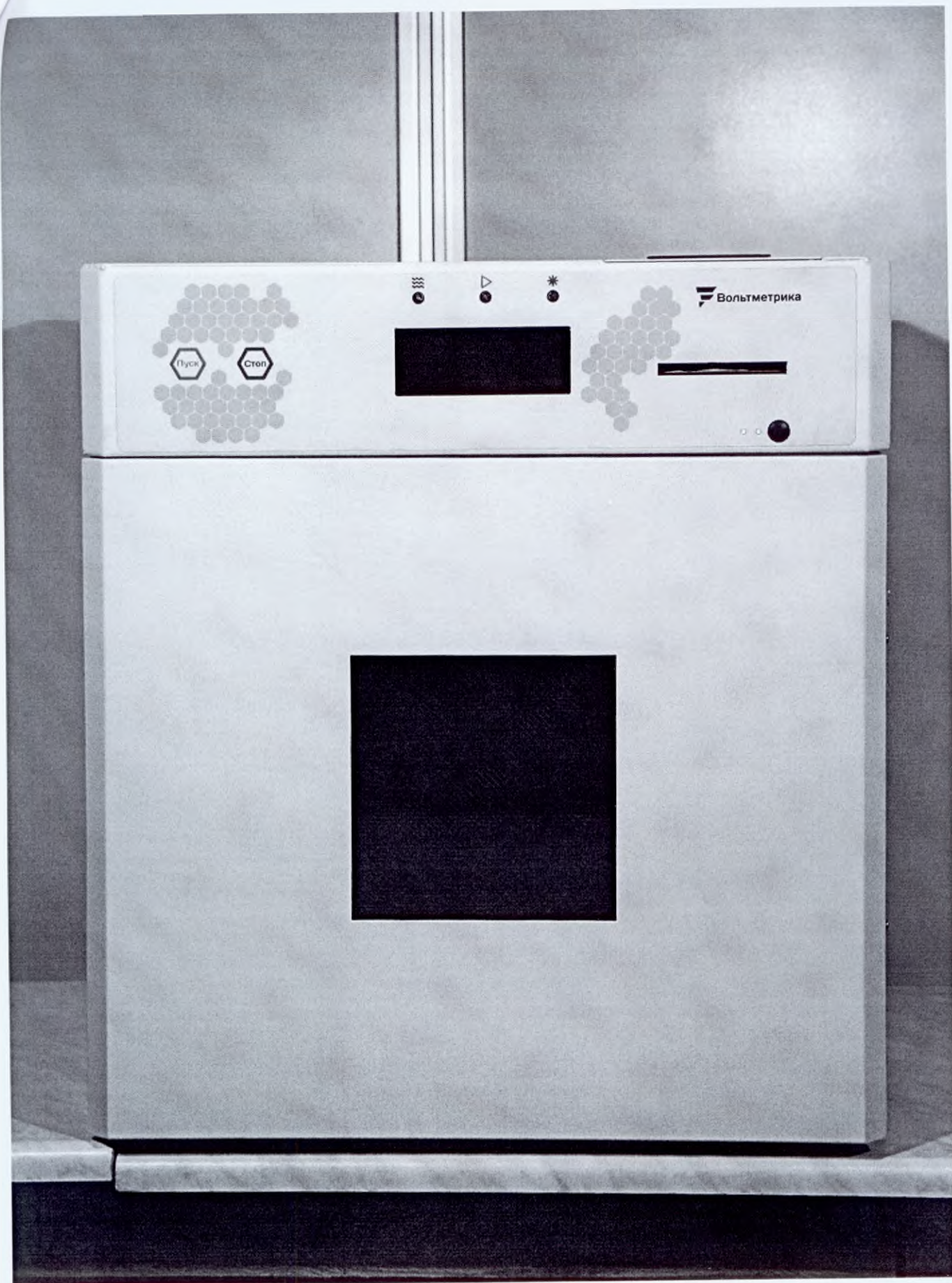
Система обеззараживания медицинских отходов микроволновая «Бионар» по ТУ 32.50.50-001-20851585-2018: Общий вид микроволновой камеры с блоком управления - Модификация 3
