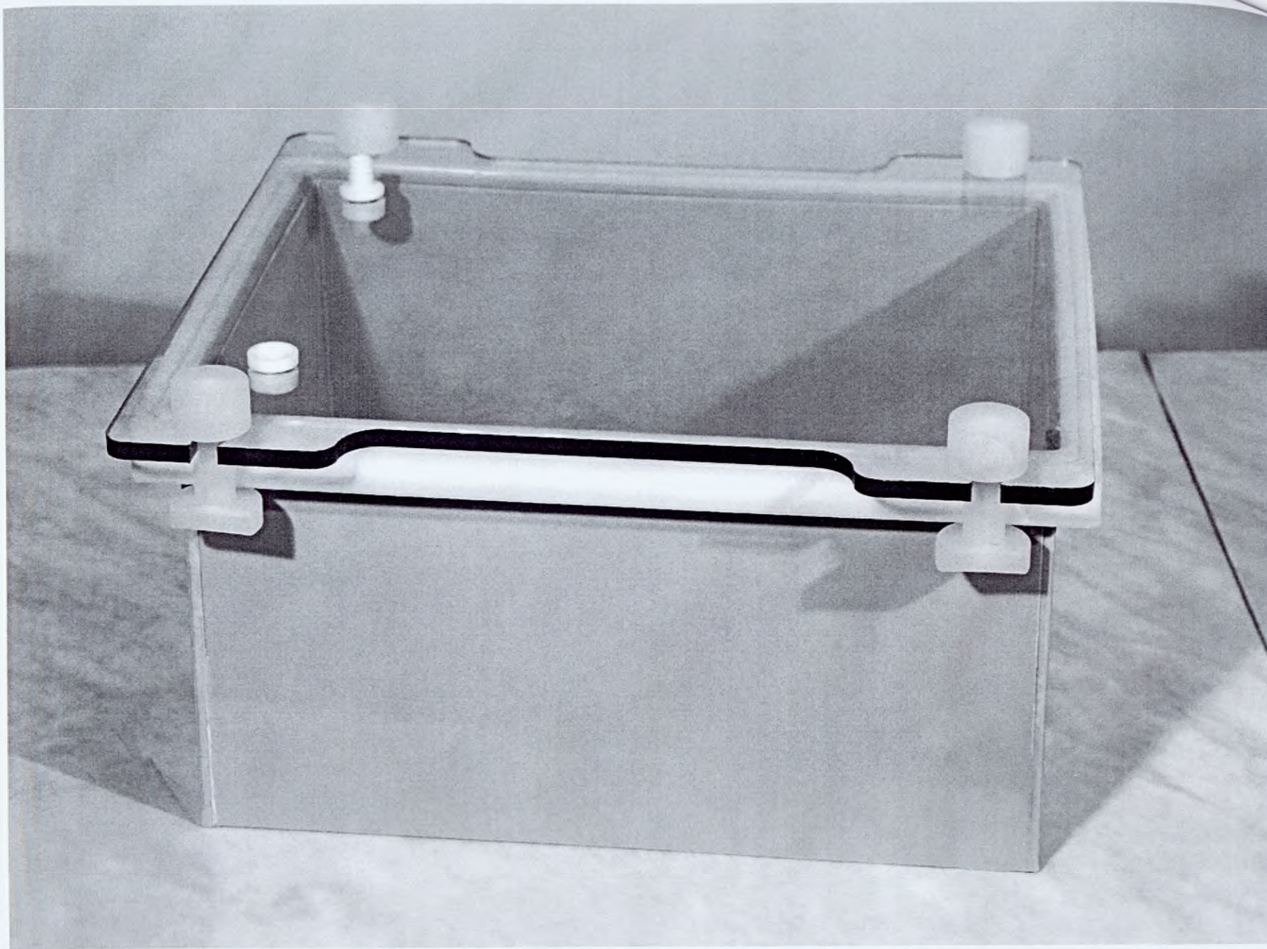
Система обеззараживания медицинских отходов микроволновая «Бионар» по ТУ 32.50.50-001-20851585-2018: Контейнер для обеззараживания - объем 4 литра
