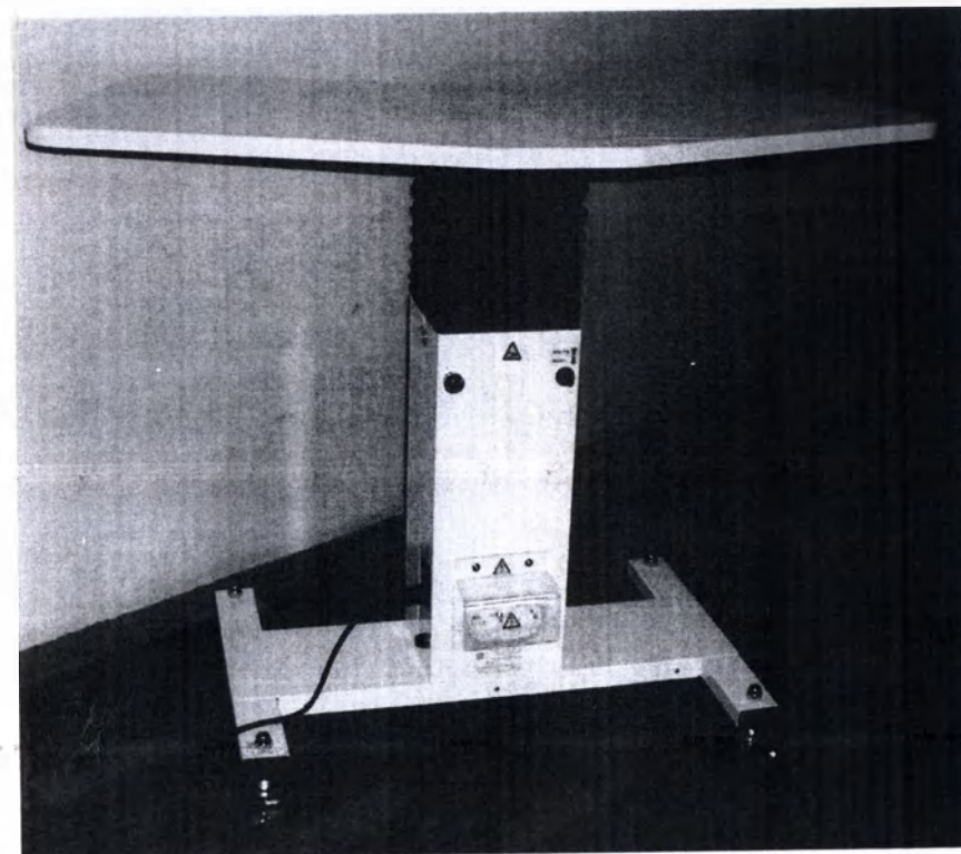
Стол медицинский с электроприводом СТЭП в различных исполнениях. Модель СТЭП-02 (исп.1) по ТУ 32.50.50-001-40307665-2017
