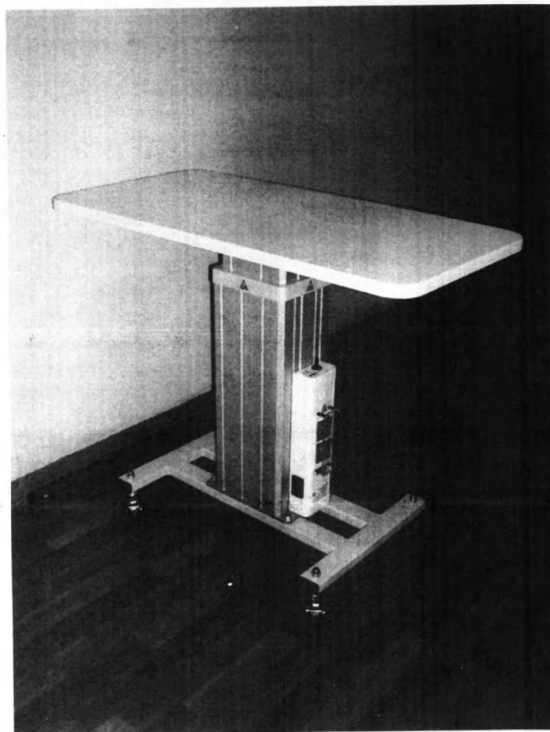
Стол медицинский с электроприводом СТЭП в различных исполнениях. Модель СТЭП-02 (исп.4) по ТУ 32.50.50-001-40307665-2017
