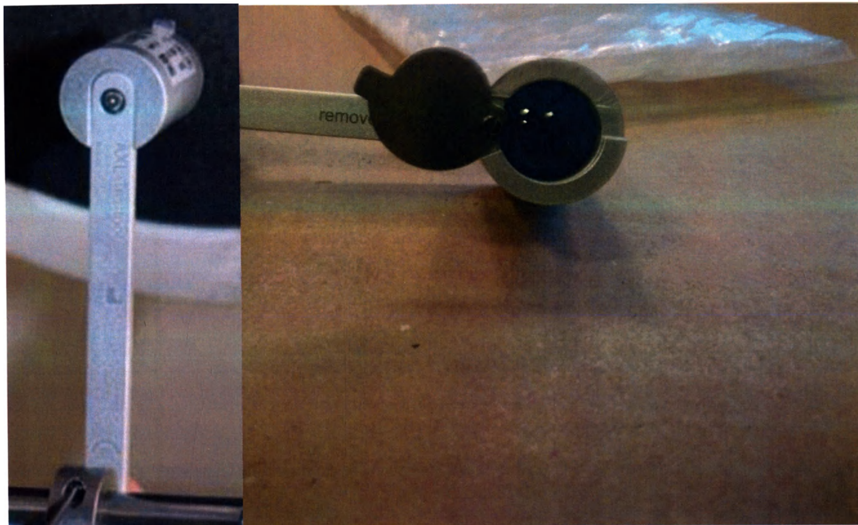
Рисунок 6 – Тестовый глаз.
