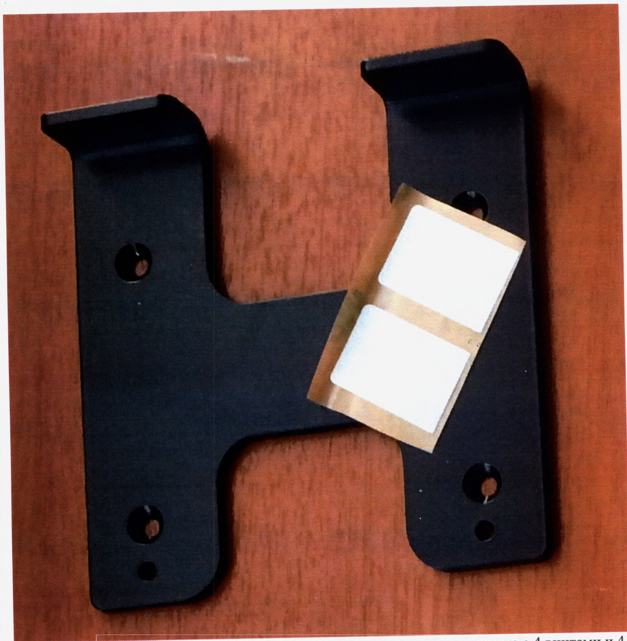
Рисунок 4 – Металлическая пластина для настенного монтажа с 4 винтами и 4 роллагами (при необходимости).
