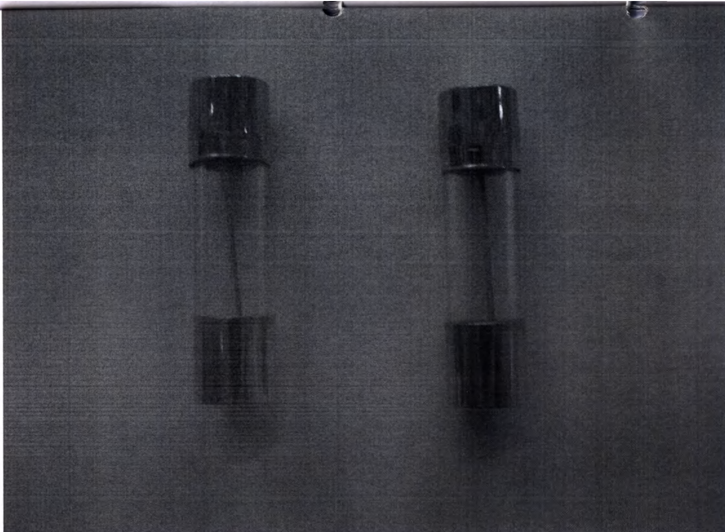
Рис.8 Вставка плавкая 5х20 10А
