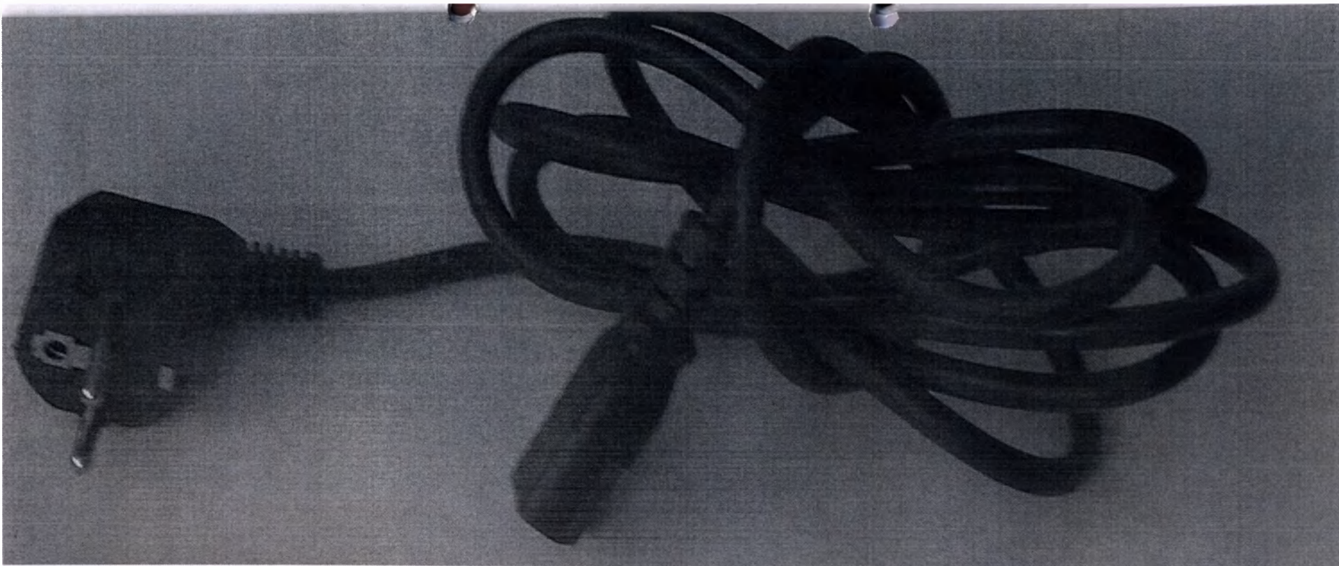
Рис.14 Кабель питания 4.5 метра, 3 \times 0.75 \text{ мм}^2
