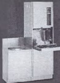
MEIKO TopLine 20 A Мощно-дезинфицирующий автомат в комплекте со специальной раковиной для настольного монтажа. Простое и компактное решение для установки мощного автомата. Размеры: ширина 1000 мм, глубина 450 мм, высота аппарата 1730 мм.
