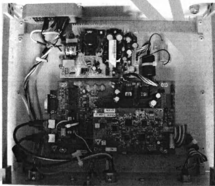
Блок видеокамеры, внутренний вид
