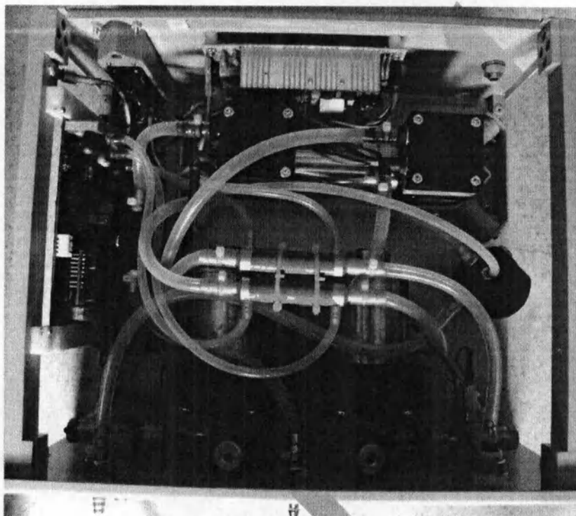
Блок газоподачи, внутренний вид
