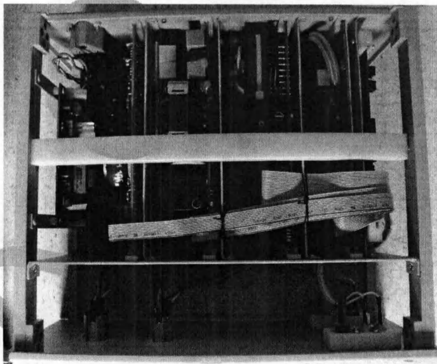
Блок ЭХВЧ, внутренний вид
