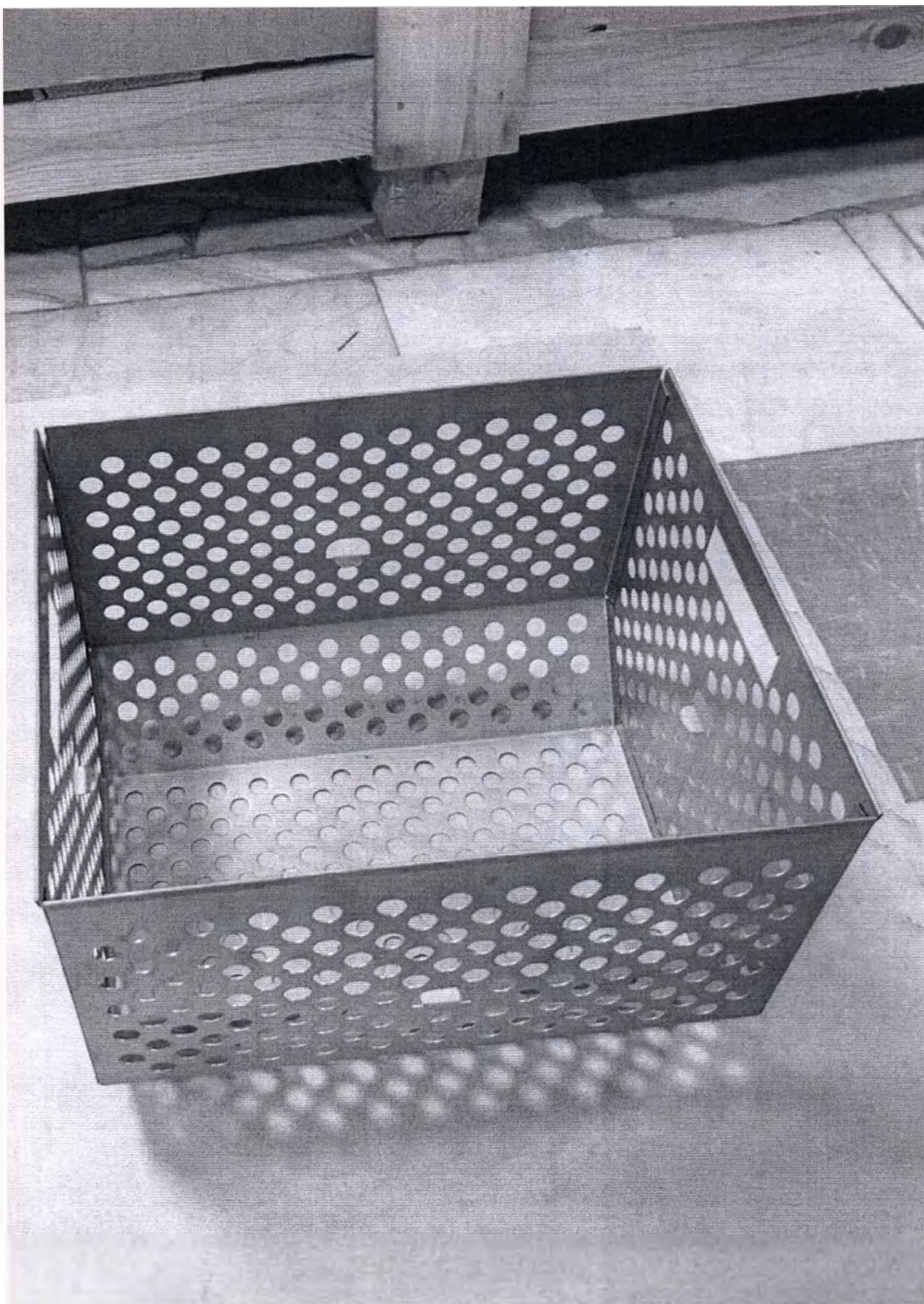
Фотографическое изображение 22. Корзина КИУС.321541.017-01
