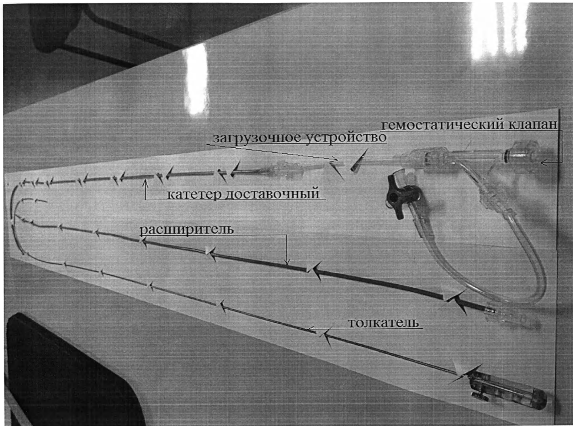
Вариант исполнения медицинского изделия: «Система транскатетерной доставки окклюдера по НАЕФ.942511.018 ТУ»: 180DS9 НАЕФ.942511.018 ТУ
