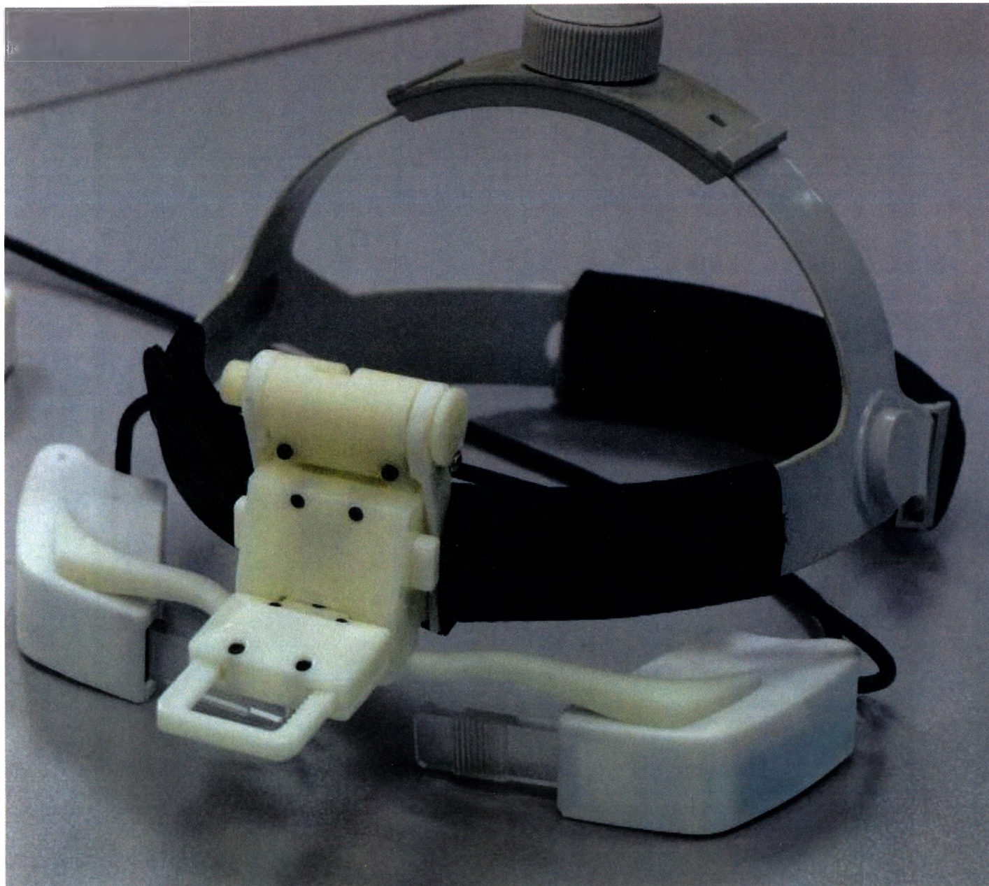
Головной блок визуализации с оголовьем
