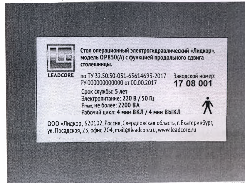
Стол операционный электрогидравлический «Лидкор», ОР850(А) с функцией продольного сдвига столешницы
