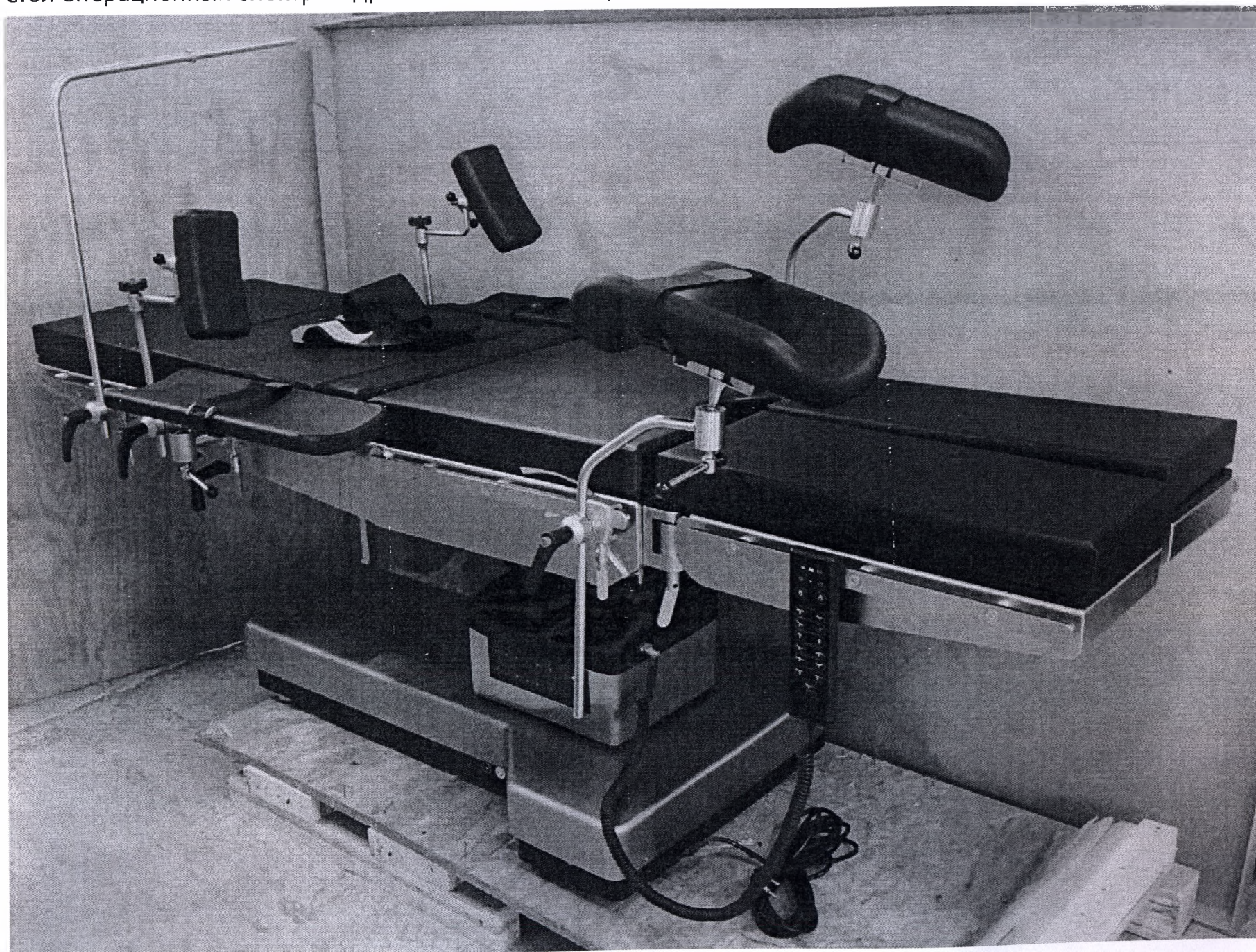
Стол операционный электрогидравлический «Лидкор», модель ОР850(А)
