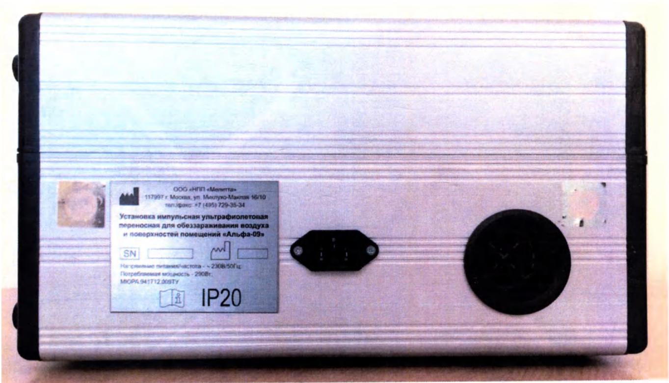
Основной блок Установки (вид слева)
