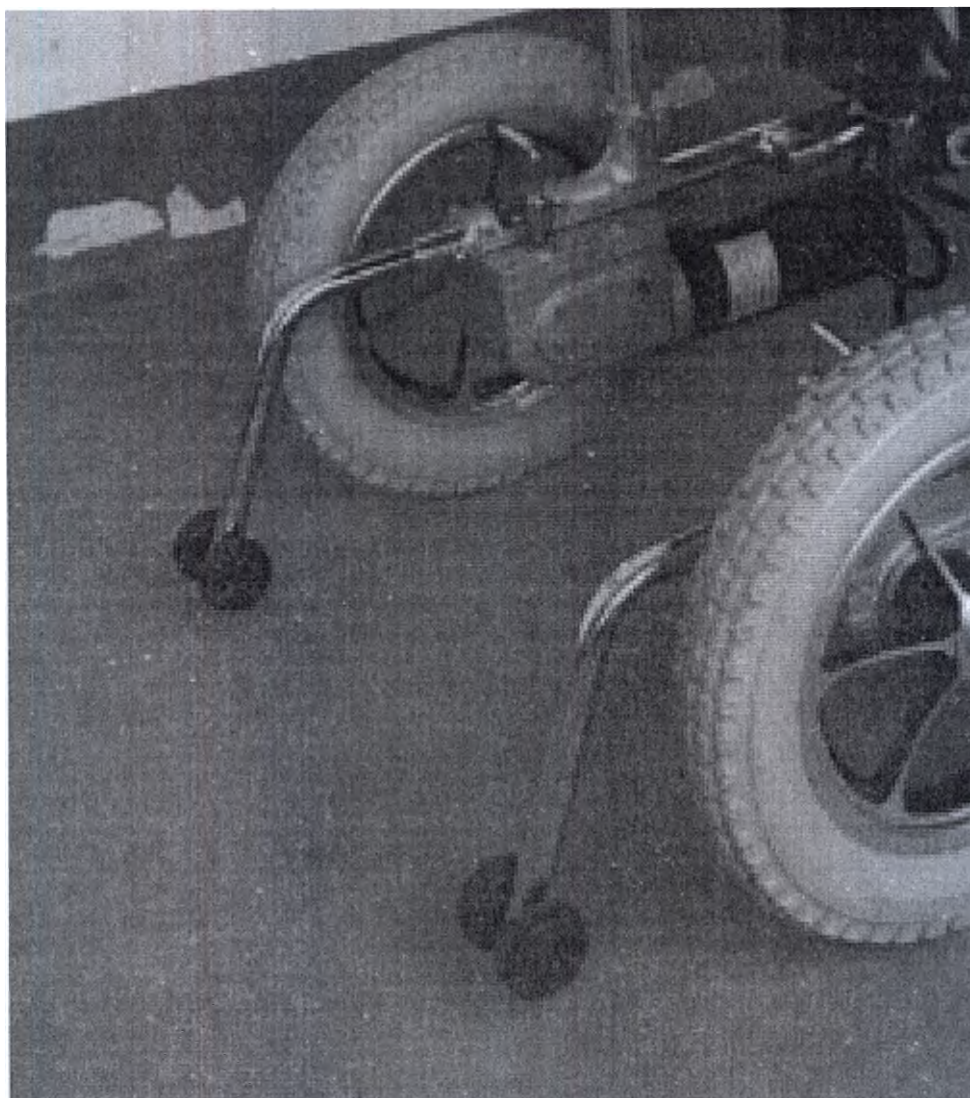
Рисунок 11 – Ролики против опрокидывания
