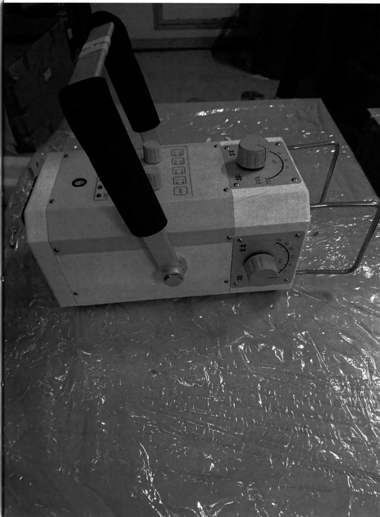
Рис.6. Рентгеновский генератор и контроллер рентгеновского излучения (моноблок) с коллиматором (Вид сбоку (слева))
