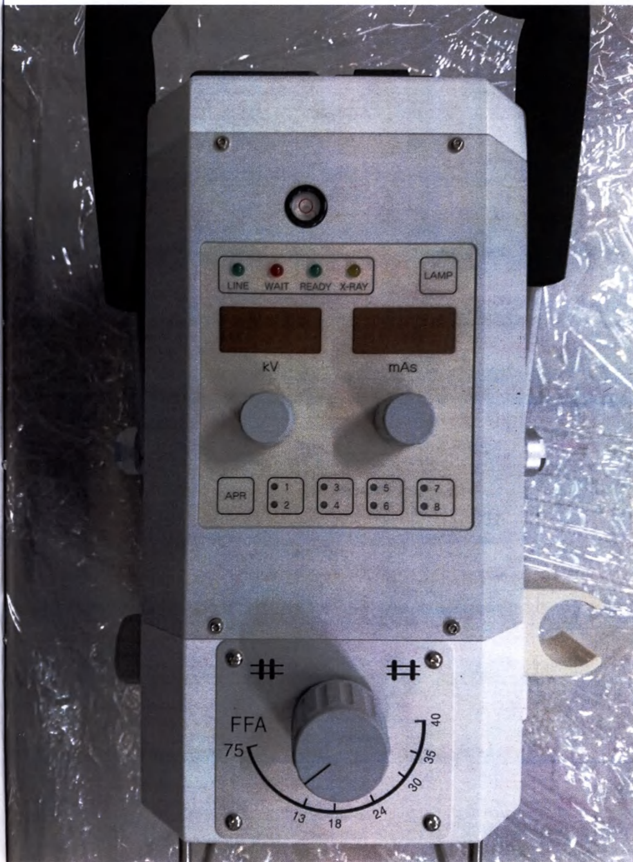
Рис.4. Рентгеновский генератор и контроллер рентгеновского излучения (моноблок) с коллиматором (вид сверху)
