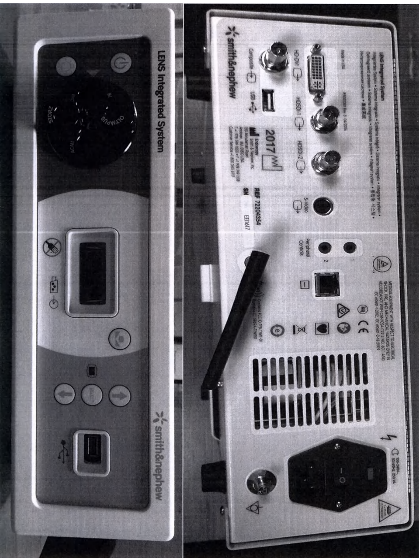
Консоль эндовидеокамеры с модулем Wi-Fi (передняя и задняя панели)
