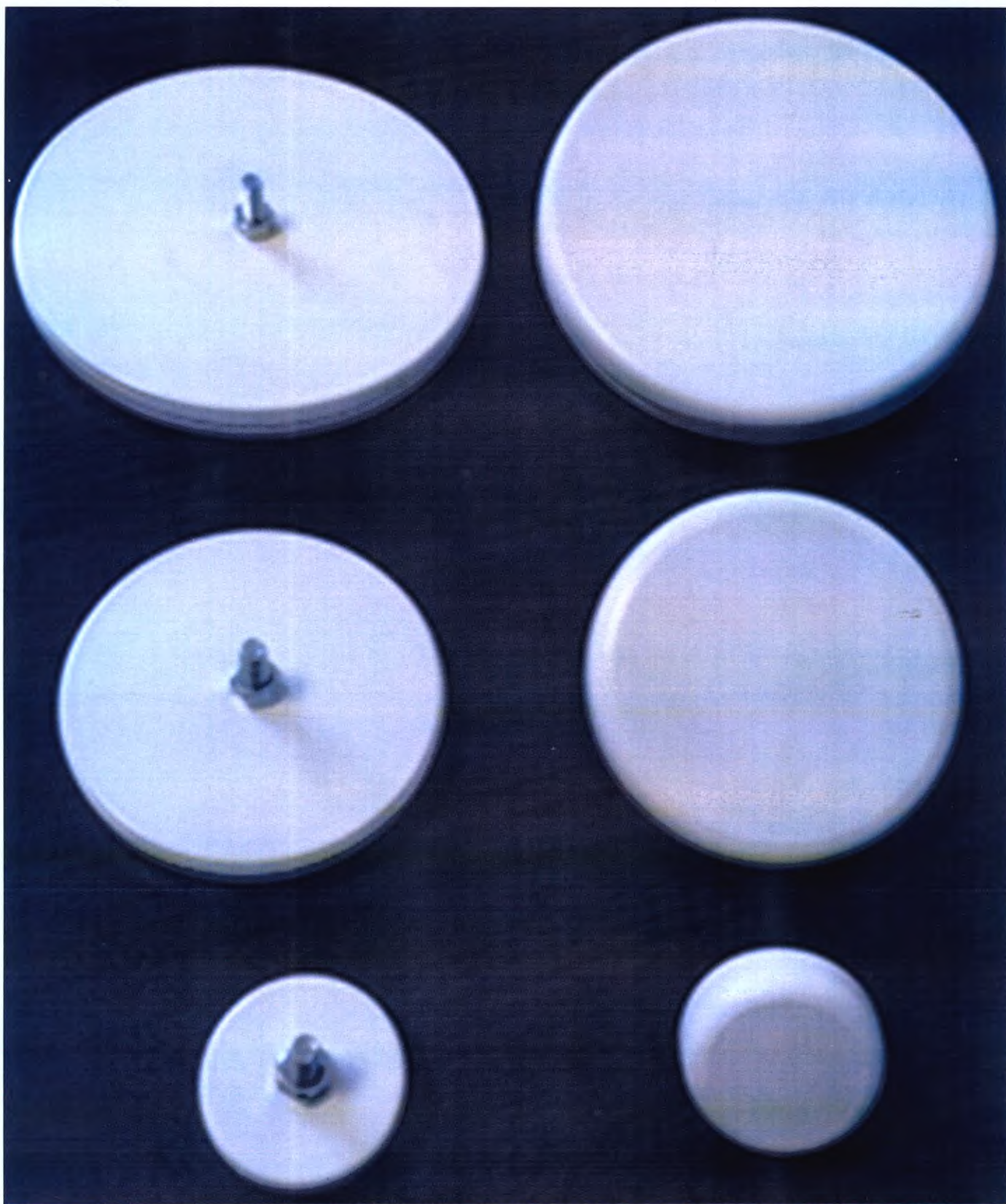
Электроды – \Phi 120, \Phi 80, \Phi 36
