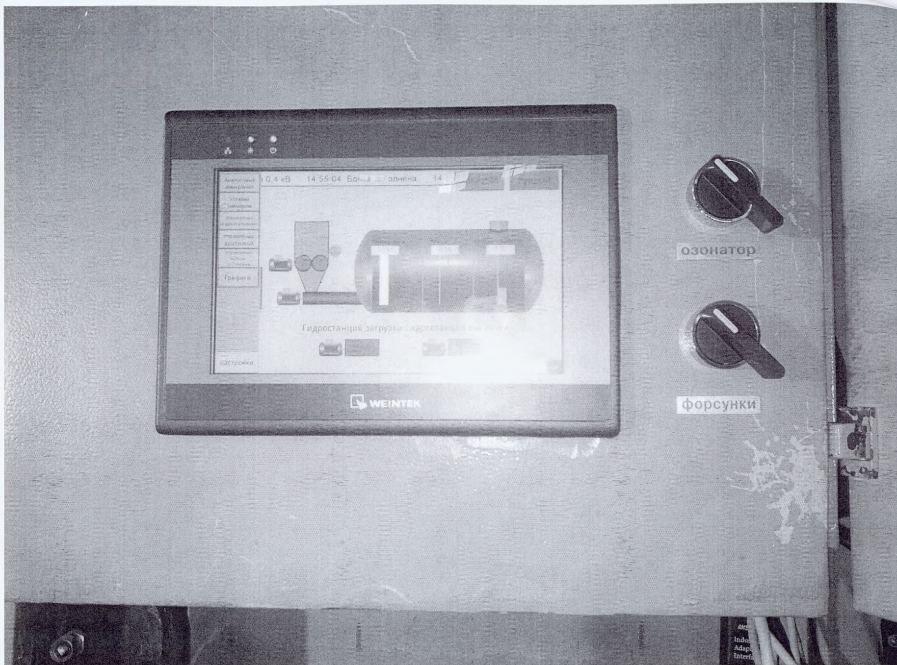
Установка мобильная по переработке и обеззараживанию медицинских отходов «ОЗСТЕР» по ТУ 32.50.50-001-05376081-2018: Программируемое контрольное устройство
