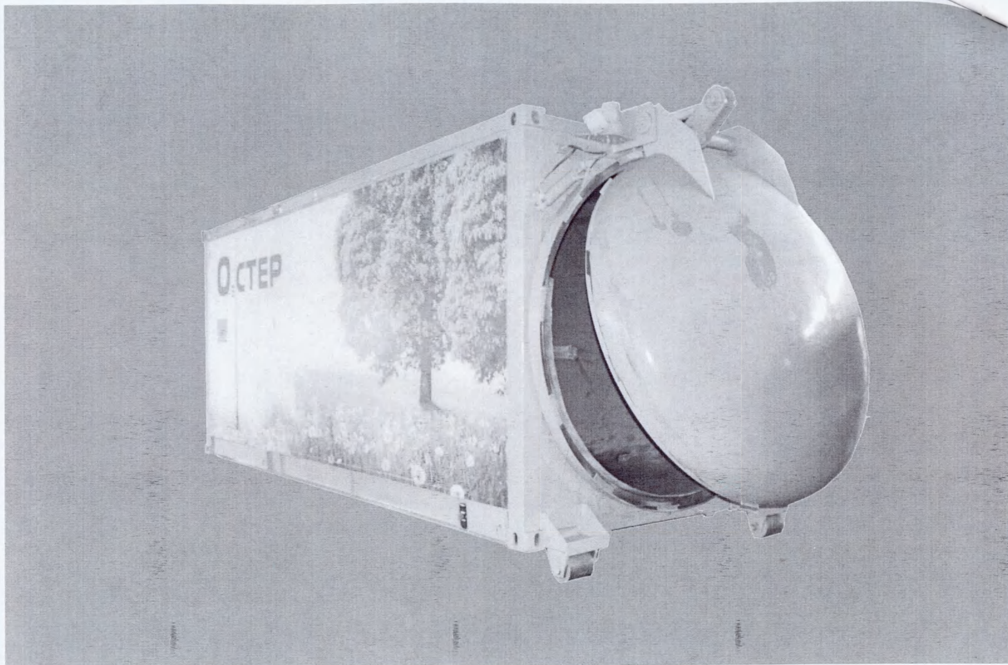
Установка мобильная по переработке и обеззараживанию медицинских отходов «О 3 СТЕР» по ТУ 32.50.50-001-05376081-2018: Общий вид установки
