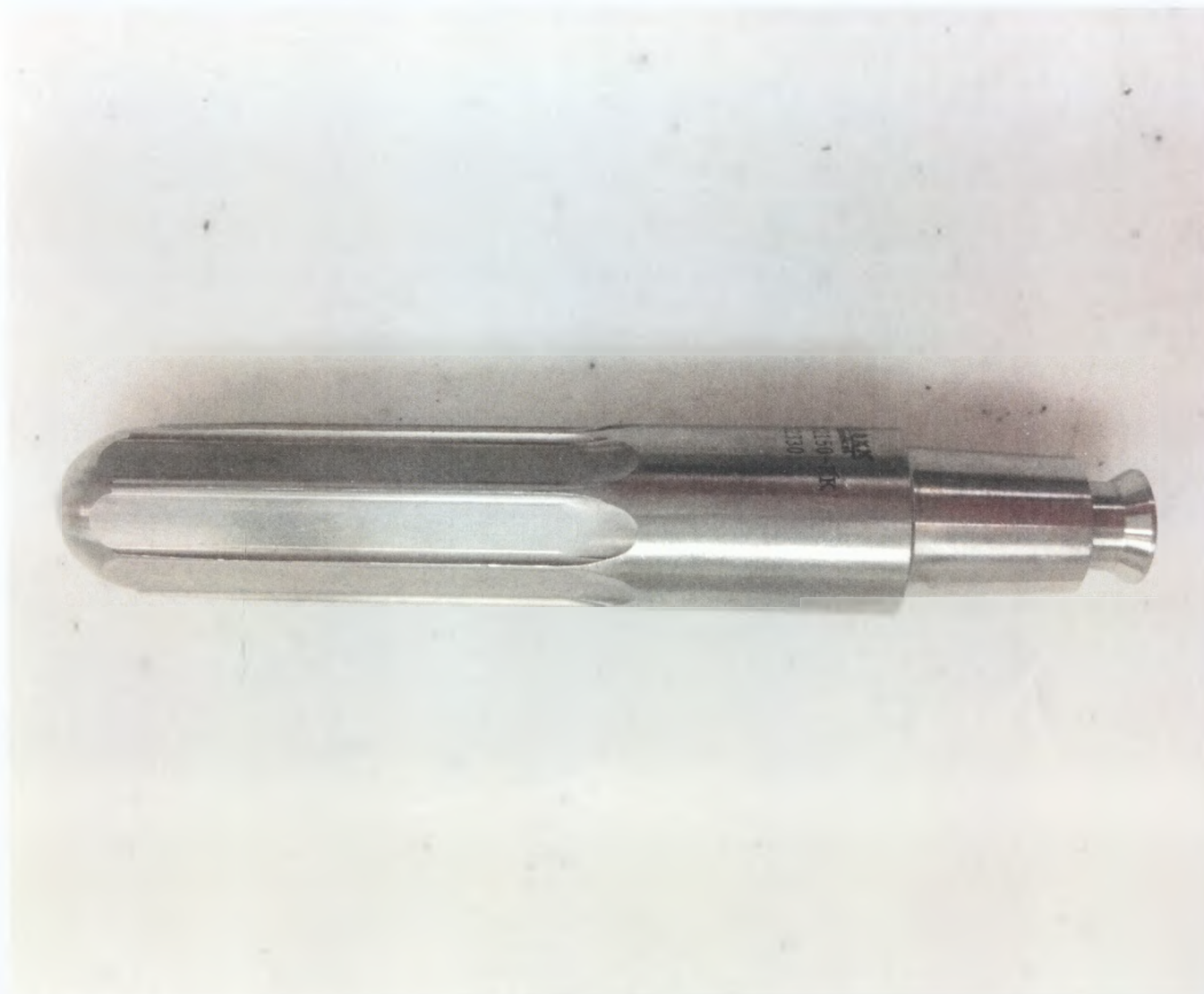
Рис.17.Удлинитель ножки эндопротеза Freedom Total Knee System (Stem Extension): RSUU2075-RK, RSUU3075-RK, RSUU4075-RK, RSUU1090-RK, RSUU2090-RK, RSUU3090-RK, RSUU4090-RK, RSUU2105-RK, RSUU3105-RK, RSUU4105-RK, RSUU1120-RK, RSUU2120-RK, RSUU3120-RK, RSUU4120-RK, RSUU2135-RK, RSUU3135-RK, RSUU4135-RK, RSUU1150-RK, RSUU2150-RK, RSUU3150-RK, RSUU4150-RK, RSUU2165-RK, RSUU3165-RK, RSUU4165-RK.
