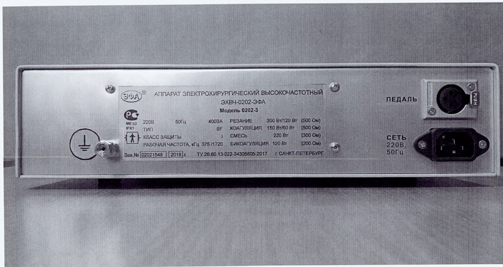
Блок ЭХВЧ ШГИЕ 941612.0202.01, модель 0202-3
