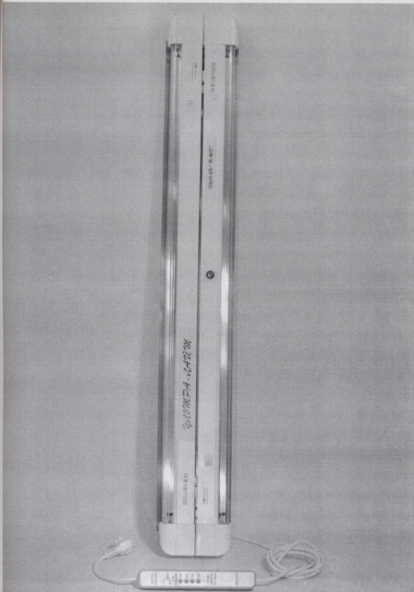
Фотография 1. Облучатель УФ-бактерицидный двухламповый настенный ОБН-05 -«Я-ФП», ТУ 9451-005-55307168-2002 (в комплектации с лампой бактерицидной типа 30 W - 2 шт.)
