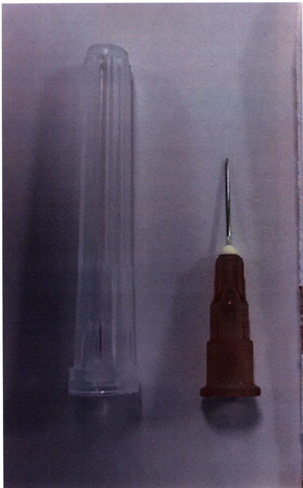
NN-2613R, наружный диаметр иглы 26G (0,45 мм), длина иглы 13 мм, длинный срез под углом 12°
