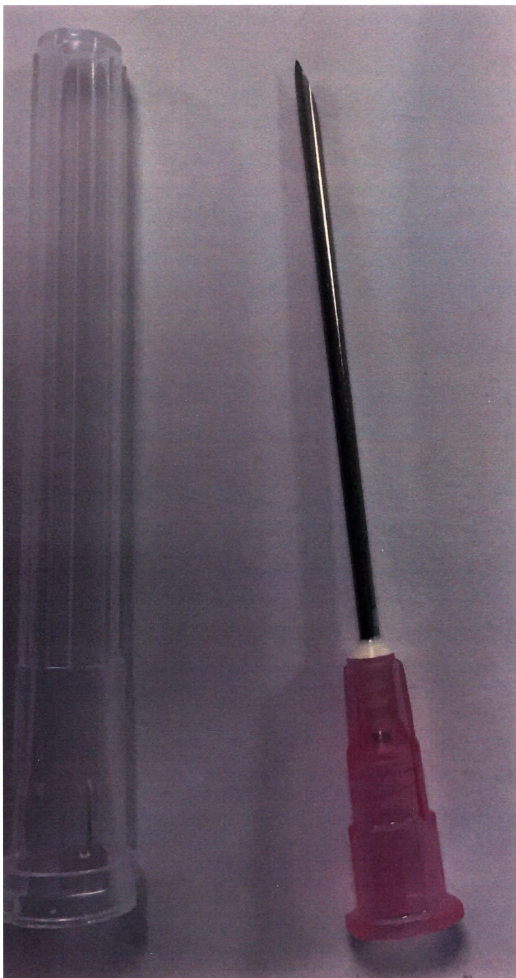
NN-1838R, наружный диаметр иглы 18G (1,2 мм), длина иглы 40 мм, длинный срез под углом 12°
