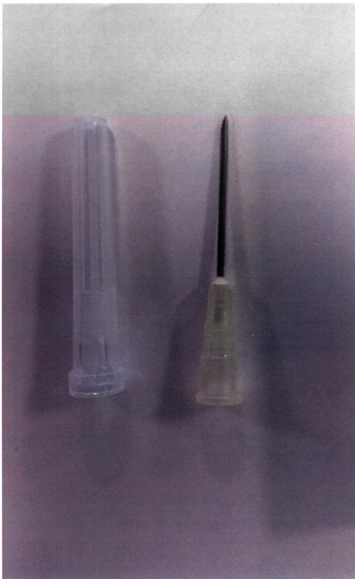
NN-1925R, наружный диаметр иглы 19G (1,1 мм), длина иглы 25 мм, длинный срез под углом 12°, (внешний вид для NN-1938R, наружный диаметр иглы 19G (1,1 мм), длина иглы 40 мм, длинный срез под углом 12° идентичен, отличие только в длине иглы)
