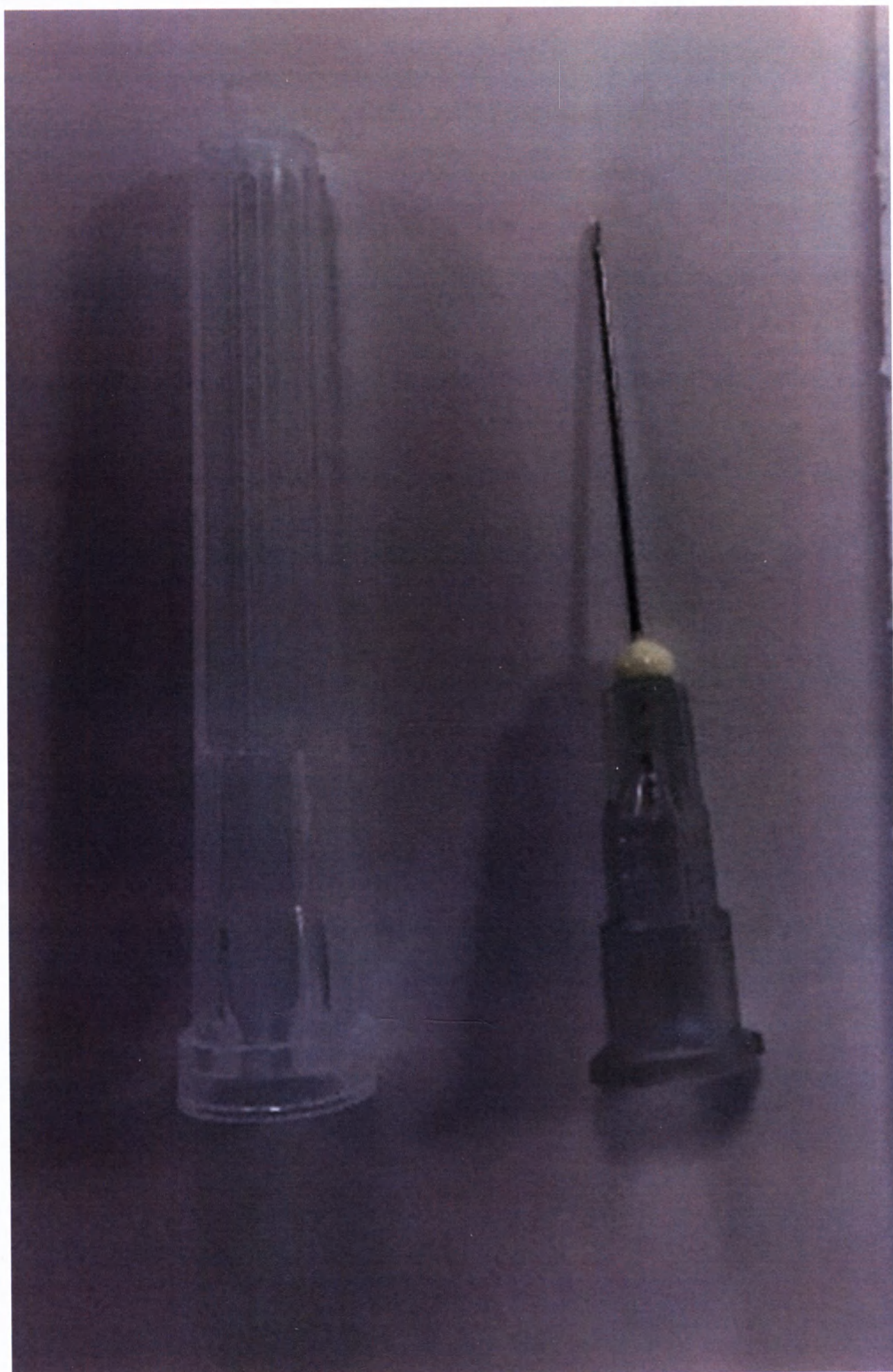
NN-2719R, наружный диаметр иглы 27G (0,4 мм), длина иглы 20 мм, длинный срез под углом 12°
