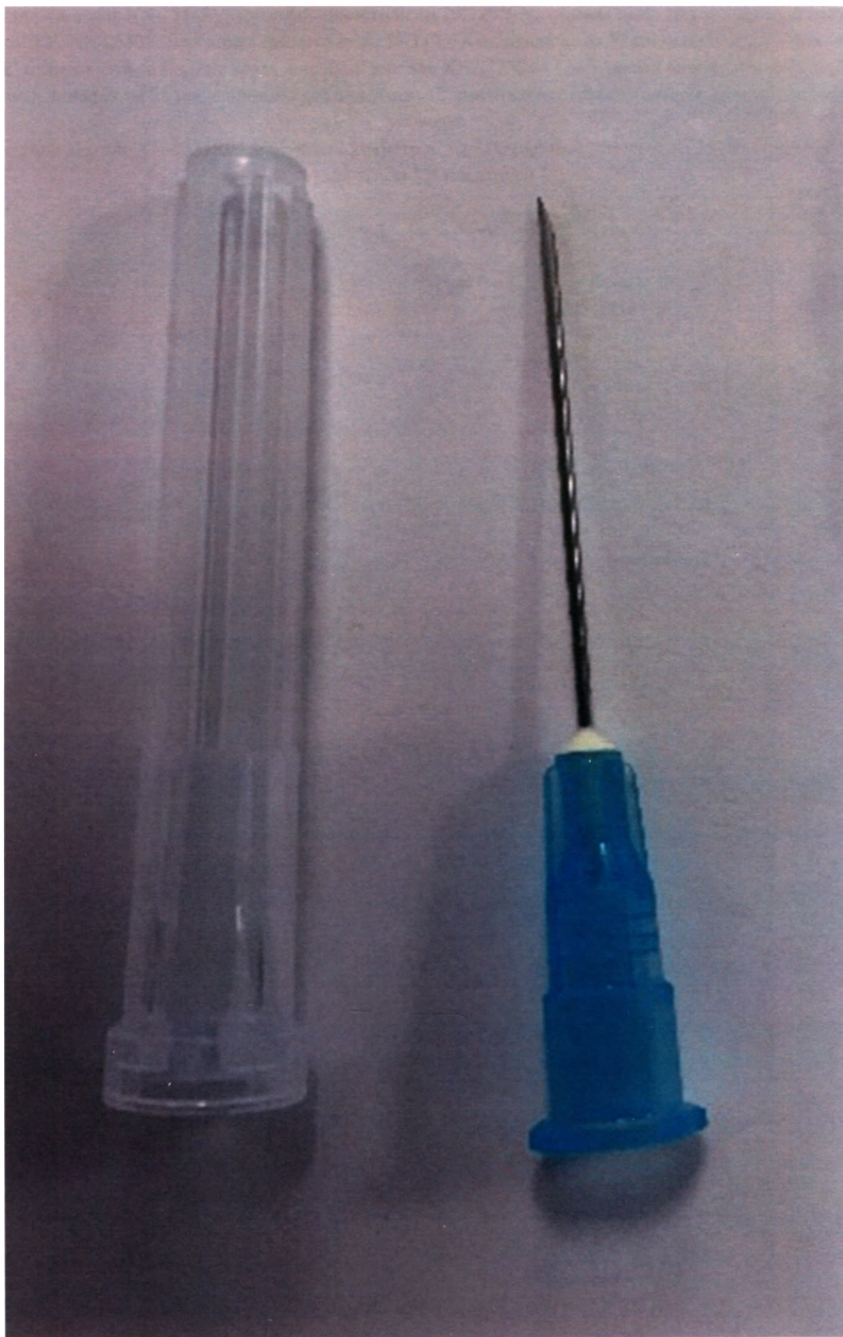
NN-2325R, наружный диаметр иглы 23G (0,6 мм), длина иглы 25 мм, длинный срез под углом 12°
