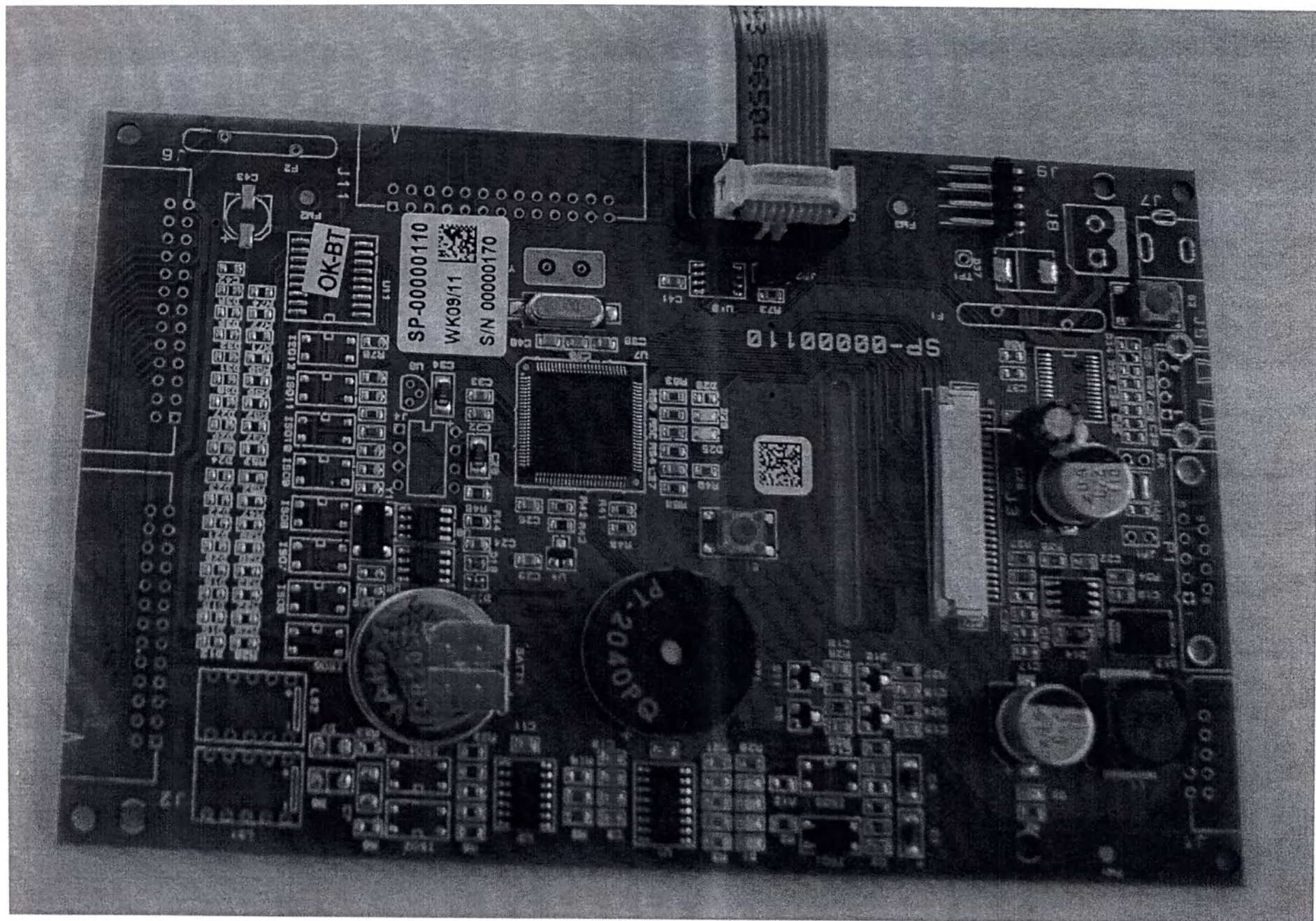
Рис. 7 - плата управления
