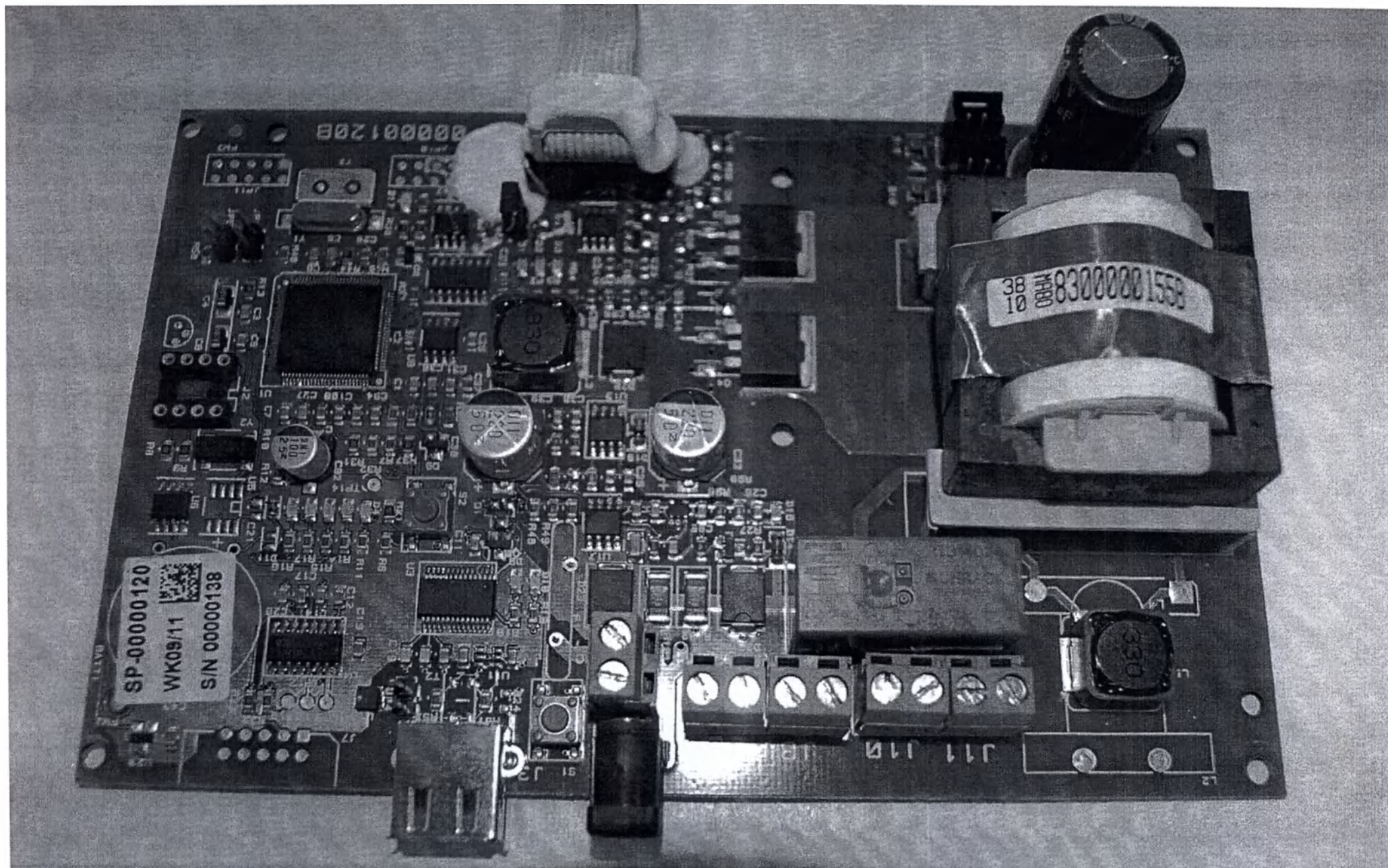
Рис. 8 - плата питания
