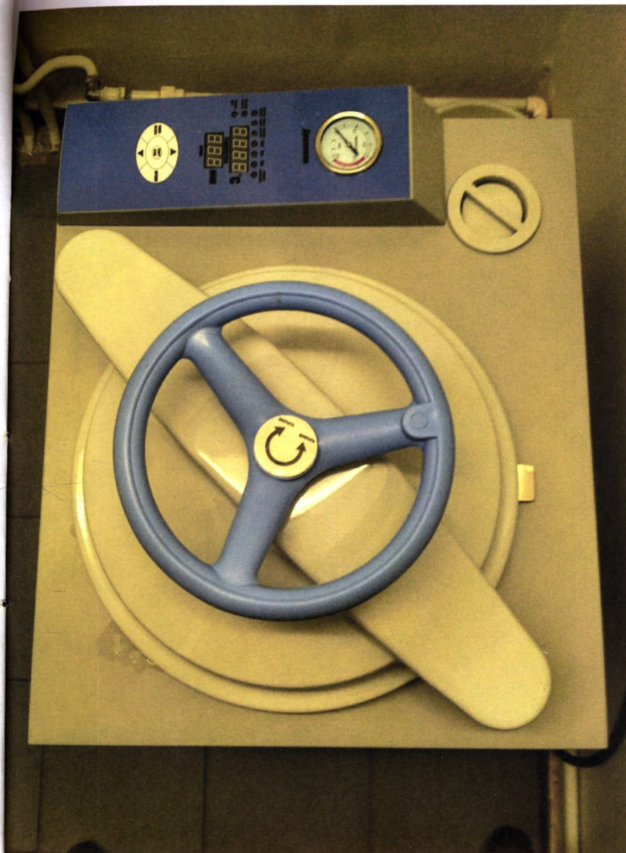
Паровой автоклав однокамерный 50 дм 3
