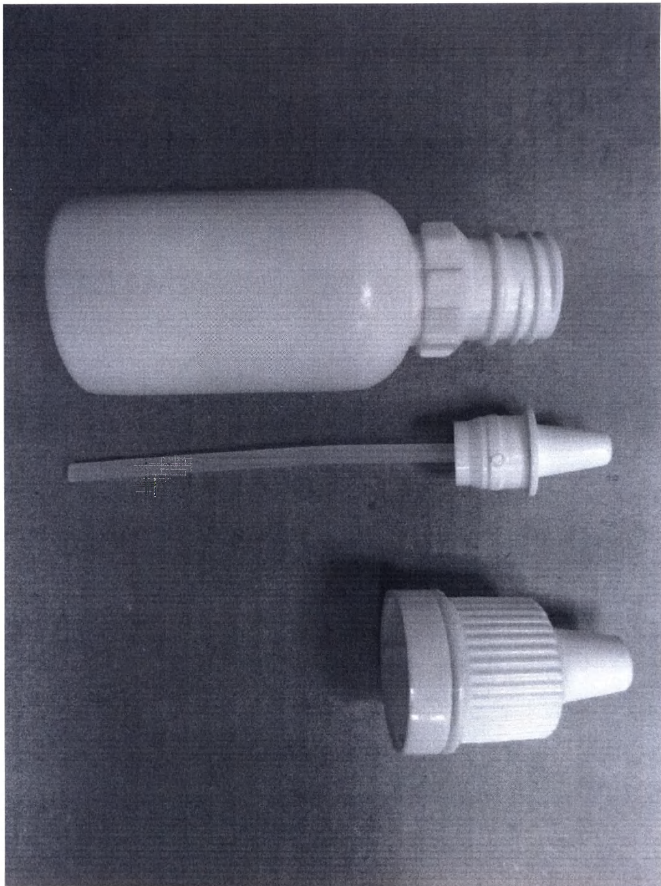
Общий вид флакона полимерного типа 1 с винтовой горловиной в комплекте с навинчиваемой крышкой с контролем первого вскрытия КНкпв14 и пробкой-капельницей ПК14.
