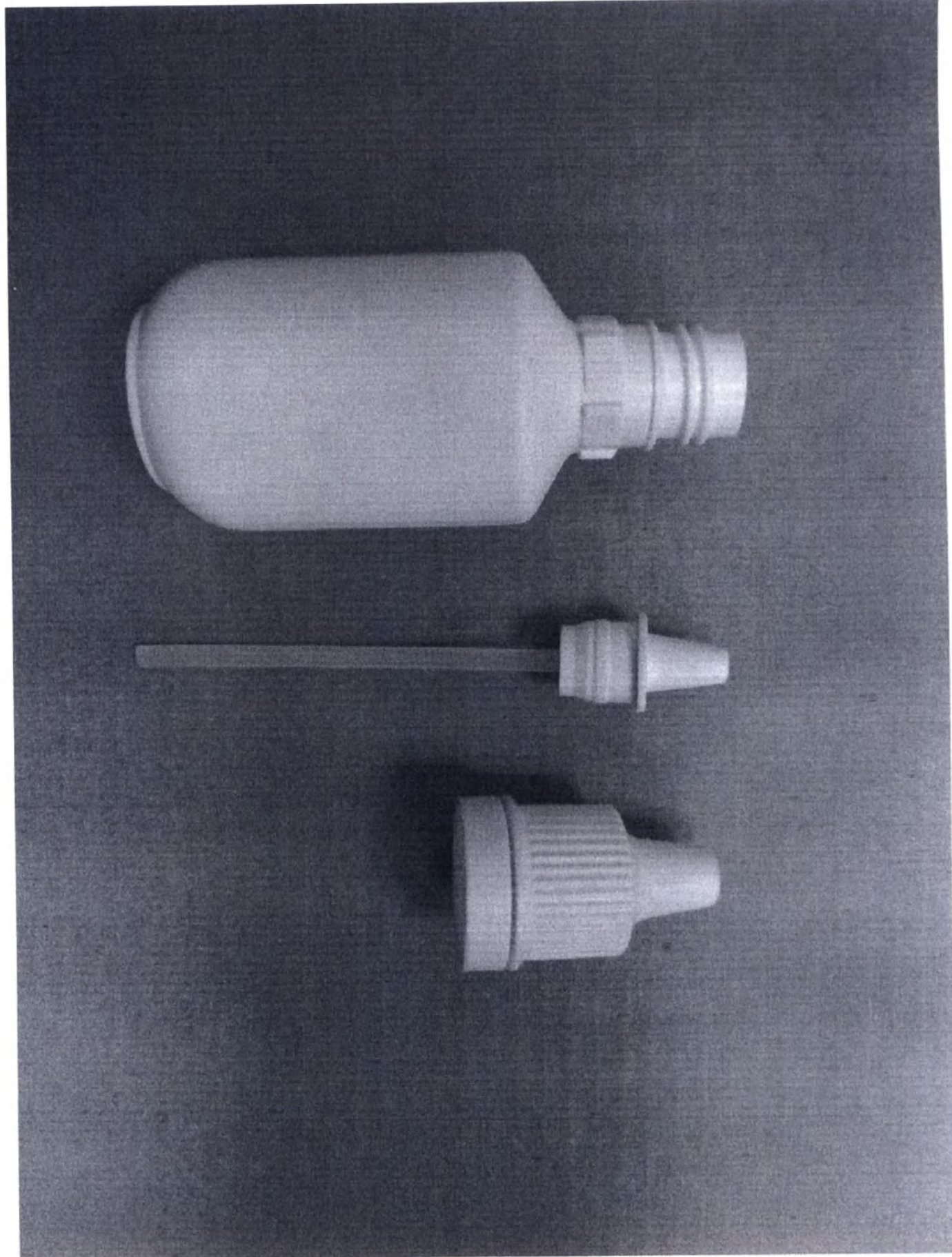
Общий вид флакона полимерного типа 2 с винтовой горловиной ФП20.14.2 объемом 20 см 3 в комплекте с навинчиваемой крышкой с контролем первого вскрытия КНкпв14 и пробкой-капельницей ПК14.
