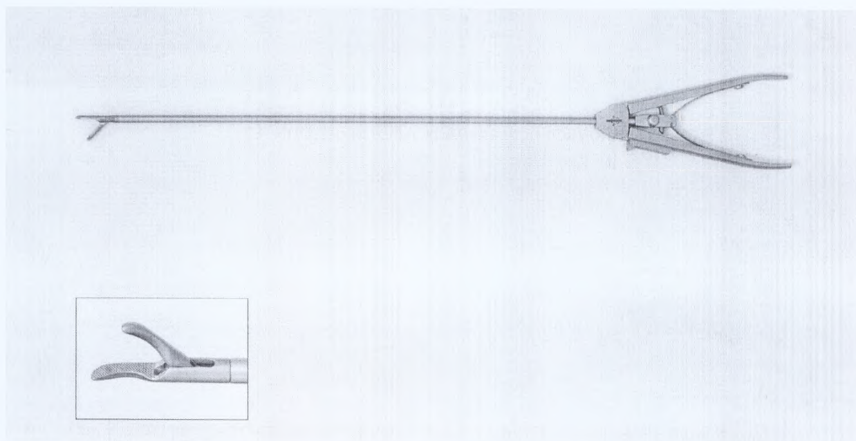
54. Иглодержатель с кремальерой изогнутый по ребру
