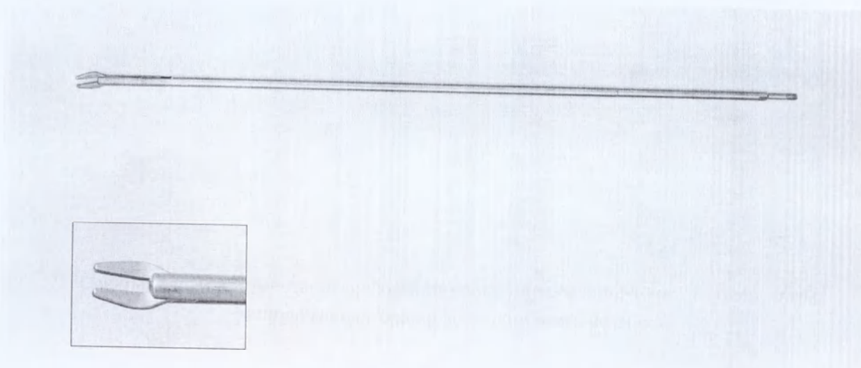
76. Сменная тяга инструмента для наложения клипс поворотного 10 мм, для клипс средне-больших
