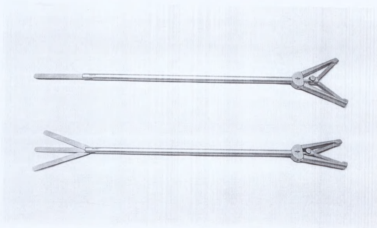
51. Ретрактор прямой 10 мм трехлепестковый
