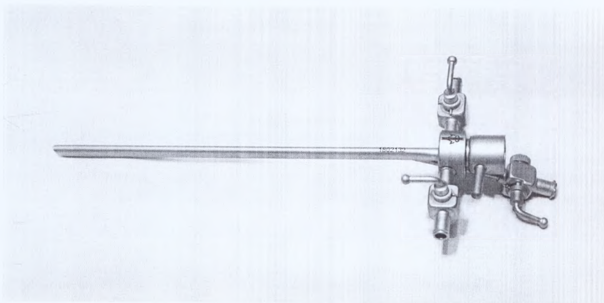
67. Тубус 14Fr (4,7 мм) с 3мм оптическим, 2 мм инструментальным и ирригационными каналами
