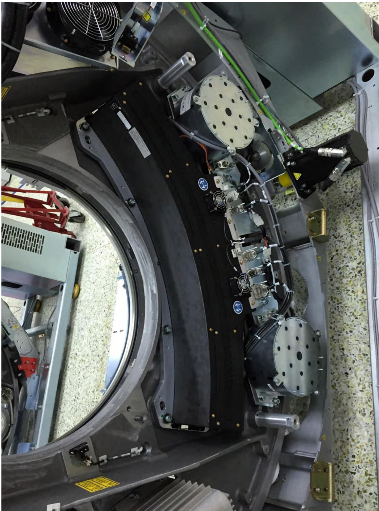
Блок детекторов
