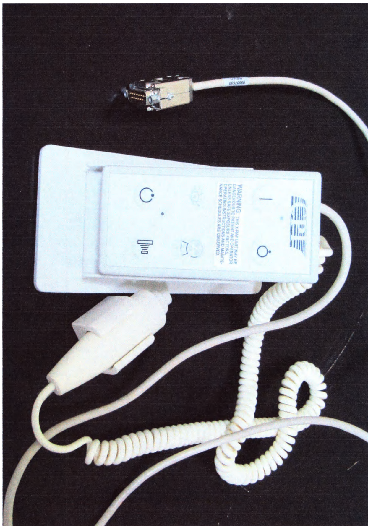
Пульт управления генераторного устройства с кнопкой включения высокого напряжения
