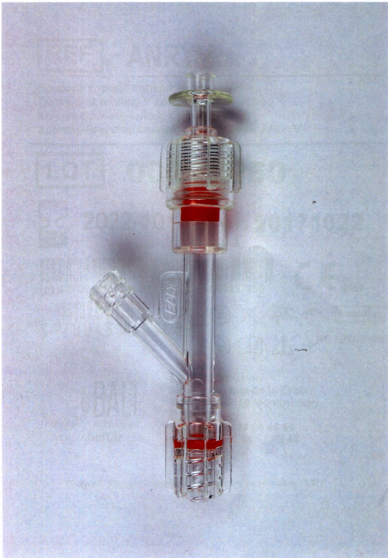
Рисунок 3. Внешний вид коннекторов Y-образных с двумя адаптерами, стерильных, одноразовых, в вариантах исполнения, RIVA.LUER, без упаковки.
