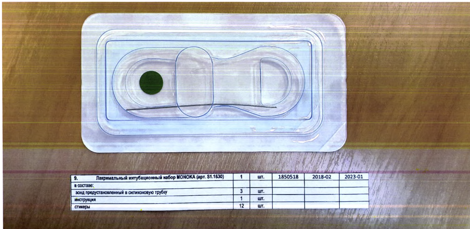
Рисунок 61 – Индивидуальная упаковка (вид спереди) арт. S1.1630
