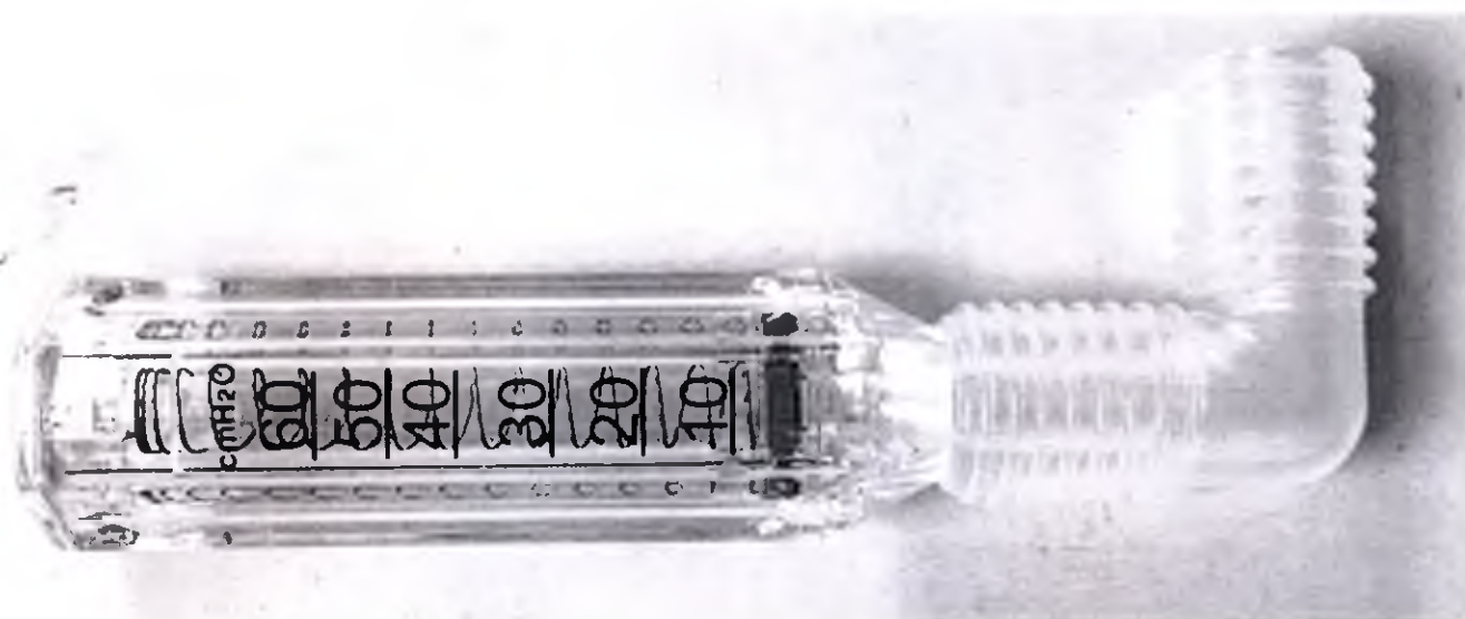
Общий вид: Манометр с угловым коннектором одноразовый.
