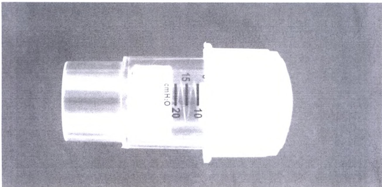
Общий вид: Клапан положительного давления на выдохе (РЕЕР-клапан) многоразовый, 0-20 см H 2 O (при необходимости).
