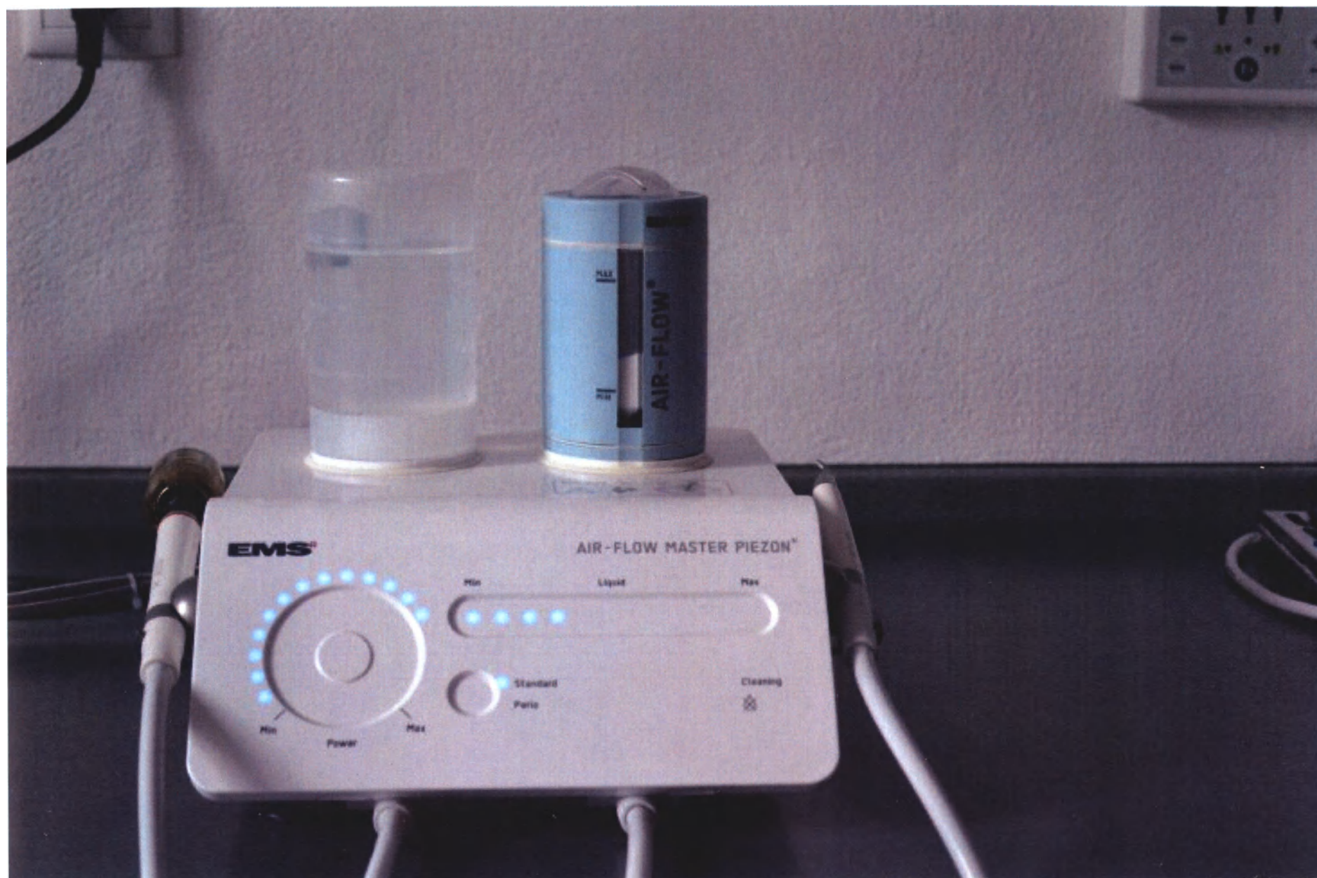
Аппарат стоматологический AIR-FLOW Master Piezon
