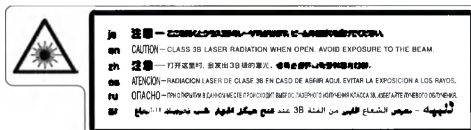
Табличка на панели о классе безопасности 3B (IEC 60825-1) (На приведенных иллюстрациях пунктиром выделена та маркировка, которая крепится изнутри устройства и не видна пользователю.)
