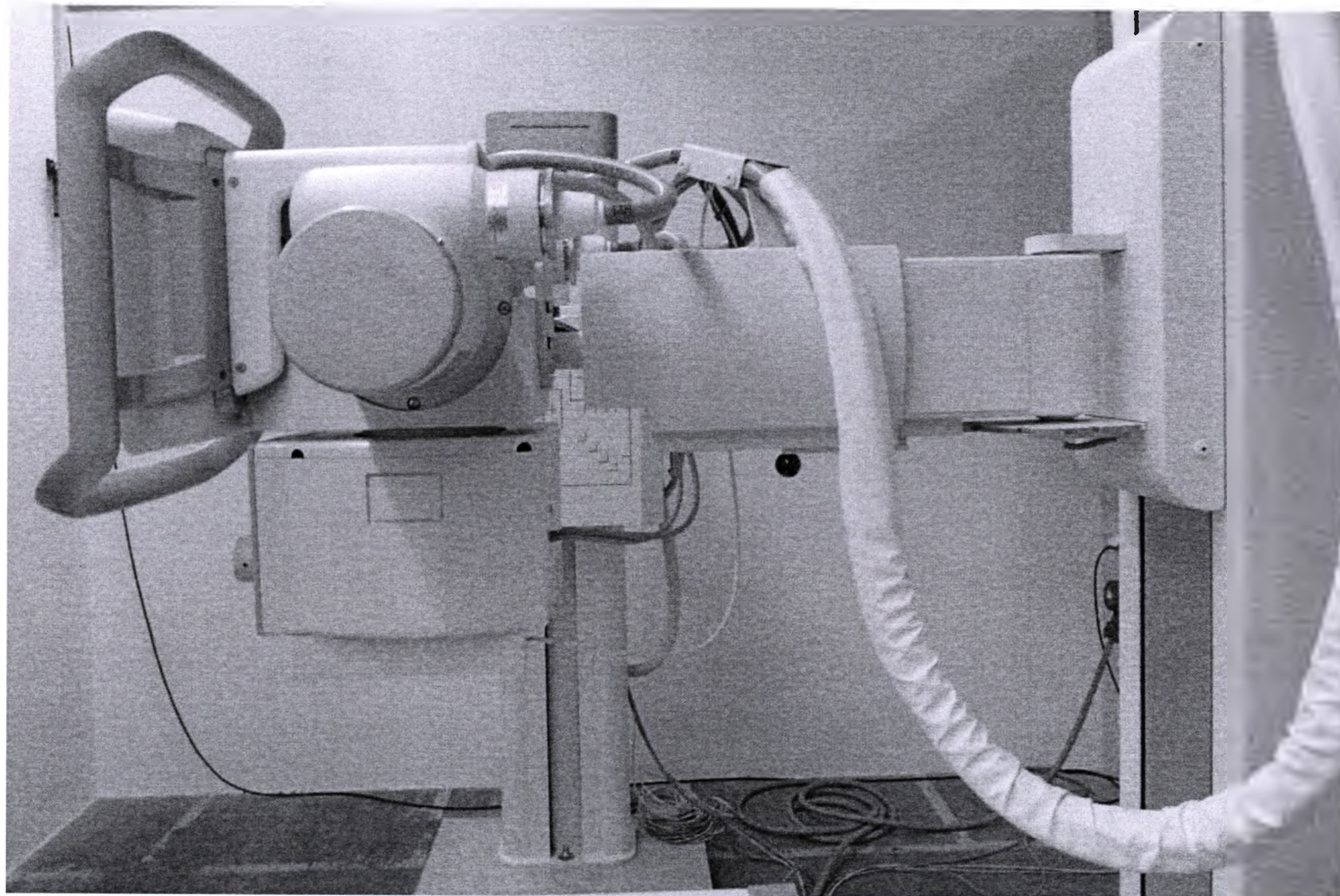
Штатив моторизированный для перемещения излучателя, напольный для DR400
