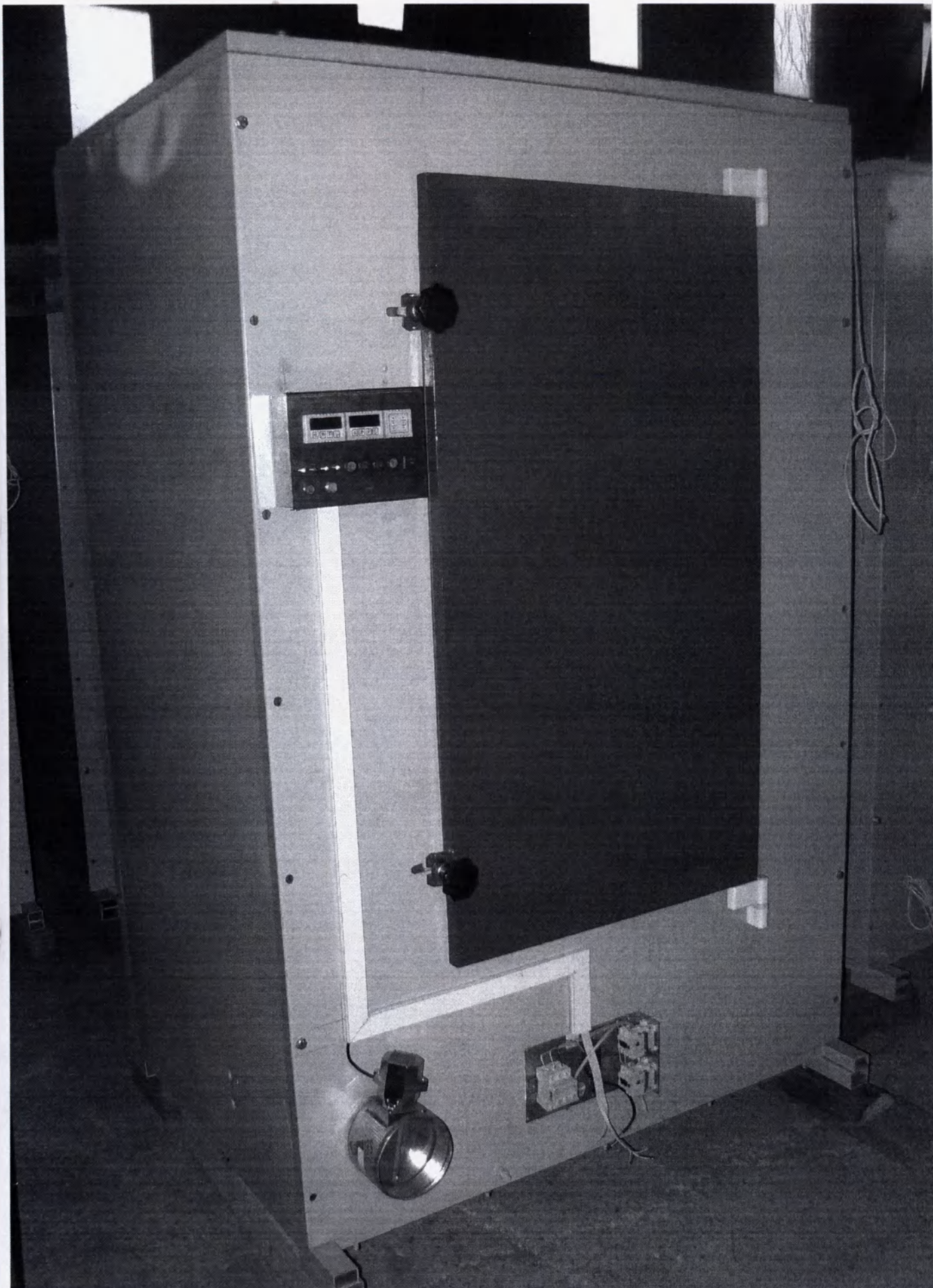
2. Камера дезинфекционная KPU-08-3 СИТИ. Изделие имеет общий вид с другими исполнениями данной группы: KPU-01-1 СИТИ, KPU-01-2 СИТИ, KPU-01-3 СИТИ, KPU-01-5 СИТИ, KPU-06-1 СИТИ, KPU-06-2 СИТИ, KPU-06-3 СИТИ, KPU-07-1 СИТИ, KPU-07-2 СИТИ, KPU-07-3 СИТИ, KPU-08-1 СИТИ, KPU-08-2 СИТИ, KPU-08-3 СИТИ. Отличие только типоразмером.
