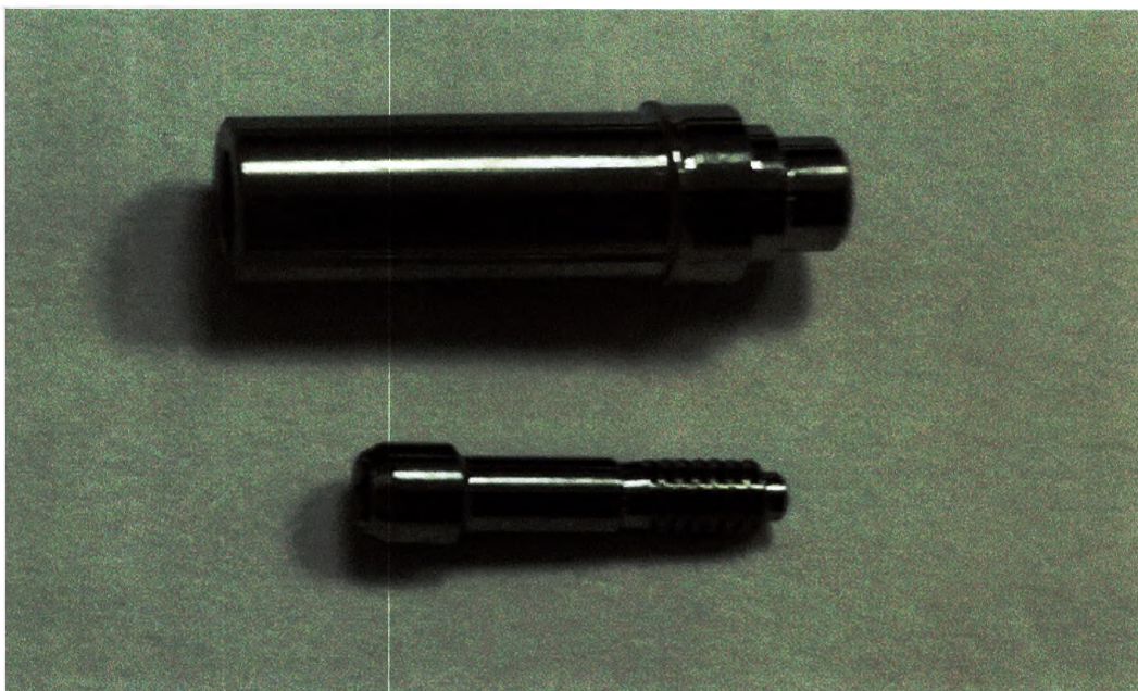
Вид Временного сварочного абатмента D3.8 XiVE® и фиксирующего винта по отдельности
