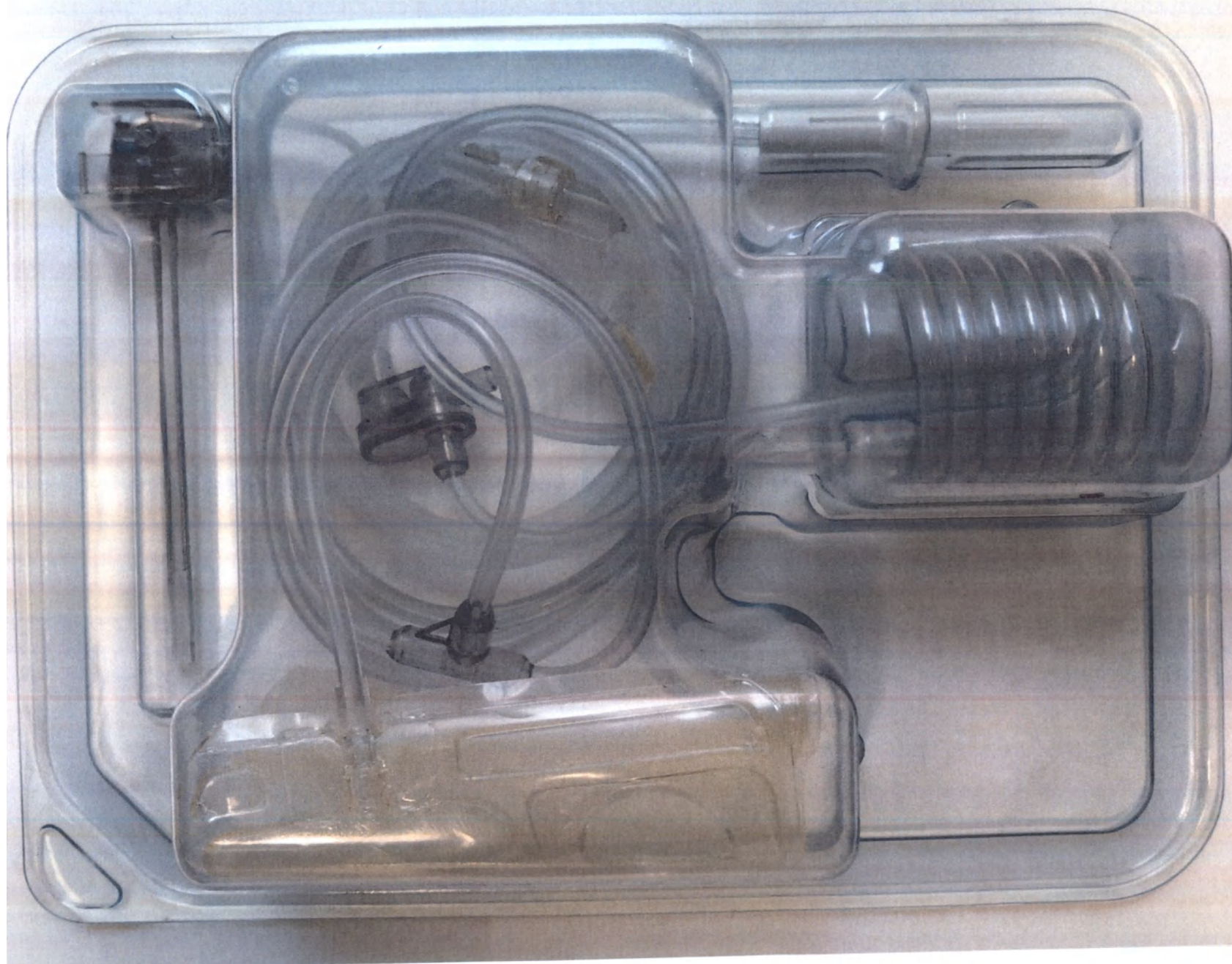
Набор одноразовый стерильный для введения источника (SAS) для системы инфузионной для позитронно-эмиссионной томографии MEDRAD
