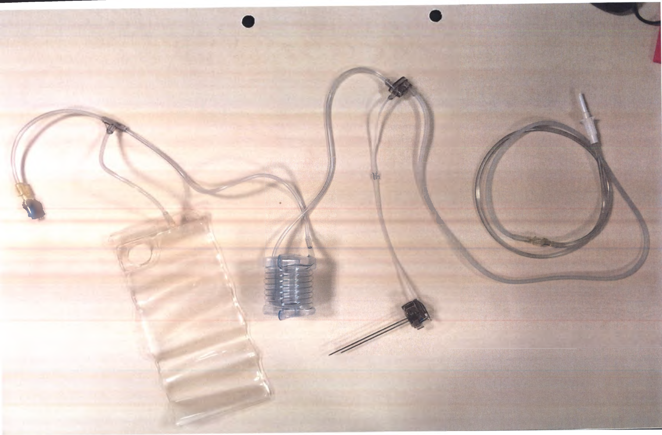
Набор одноразовый стерильный для введения источника (SAS) для системы инфузионной для позитронно-эмиссионной томографии MEDRAD Intego в составе в общем виде (без упаковки)
