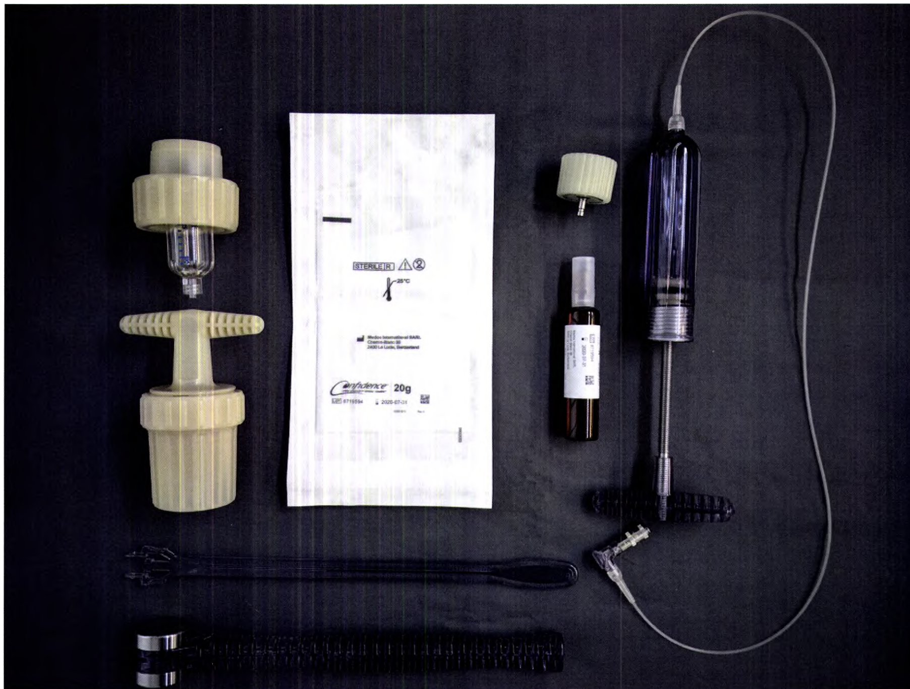
Система костного цемента Confidence повышенной вязкости, вариант исполнения: Система костного цемента Confidence повышенной вязкости, набор 11сс
