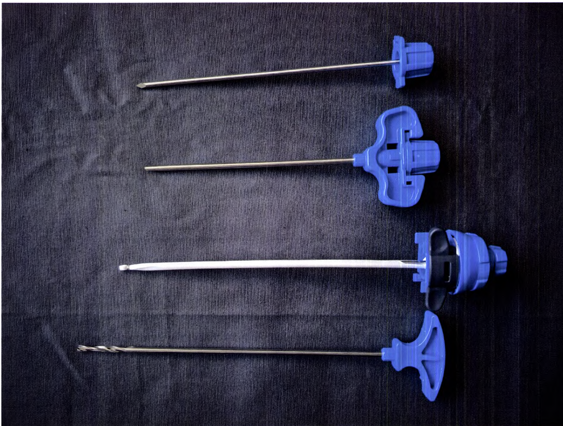
Набор принадлежностей Confidence Perimeter для введения костного цемента повышенной вязкости
