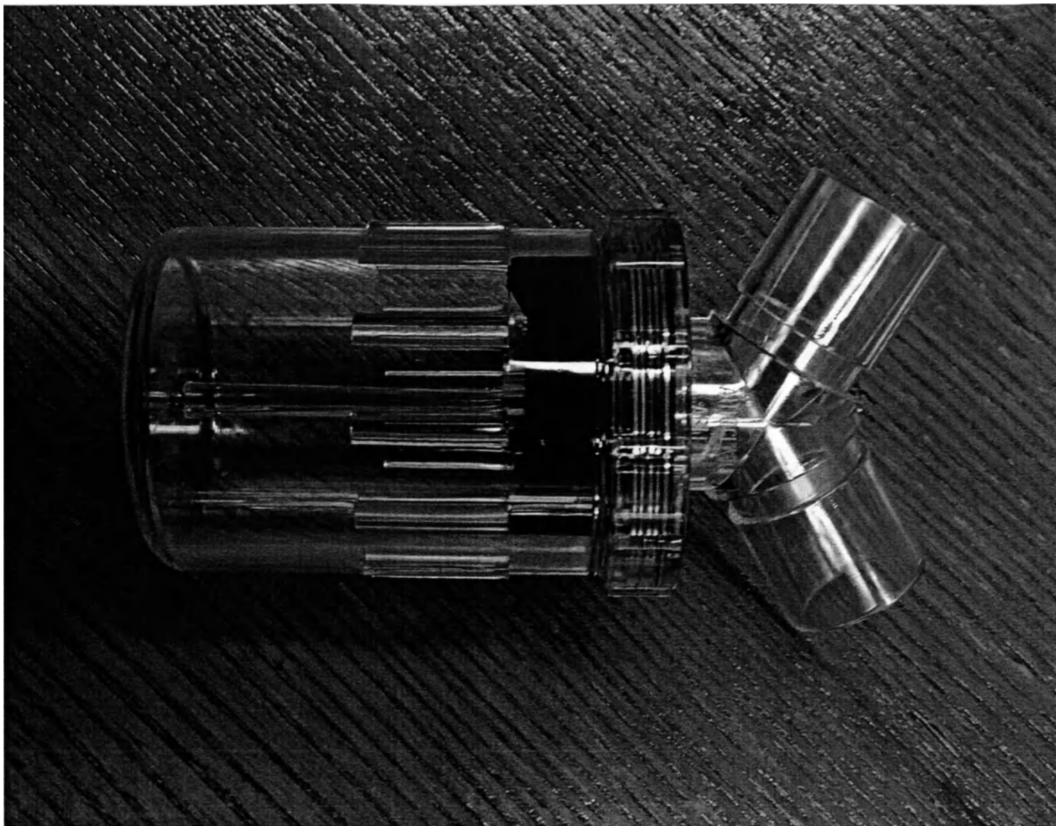
Влагосборник неонатальный
