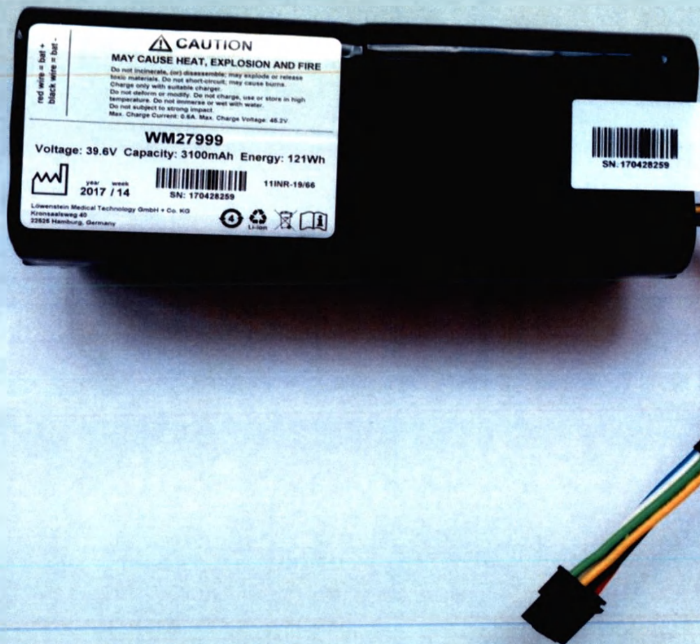
Аккумуляторная батарея
