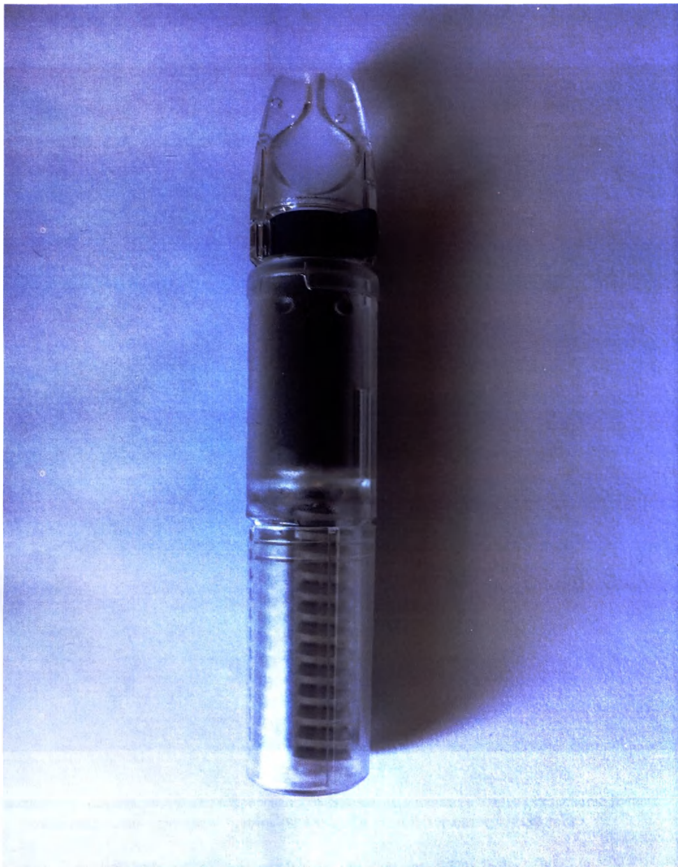
Внешний вид медицинского изделия «Устройство точного позиционирования коронарных стентов (SPAS) по ТУ 32.50.13.190-001-45929489-2018»
