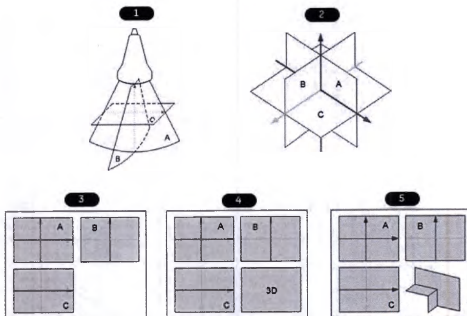
Рисунок 8-1 Плоскости сечения
