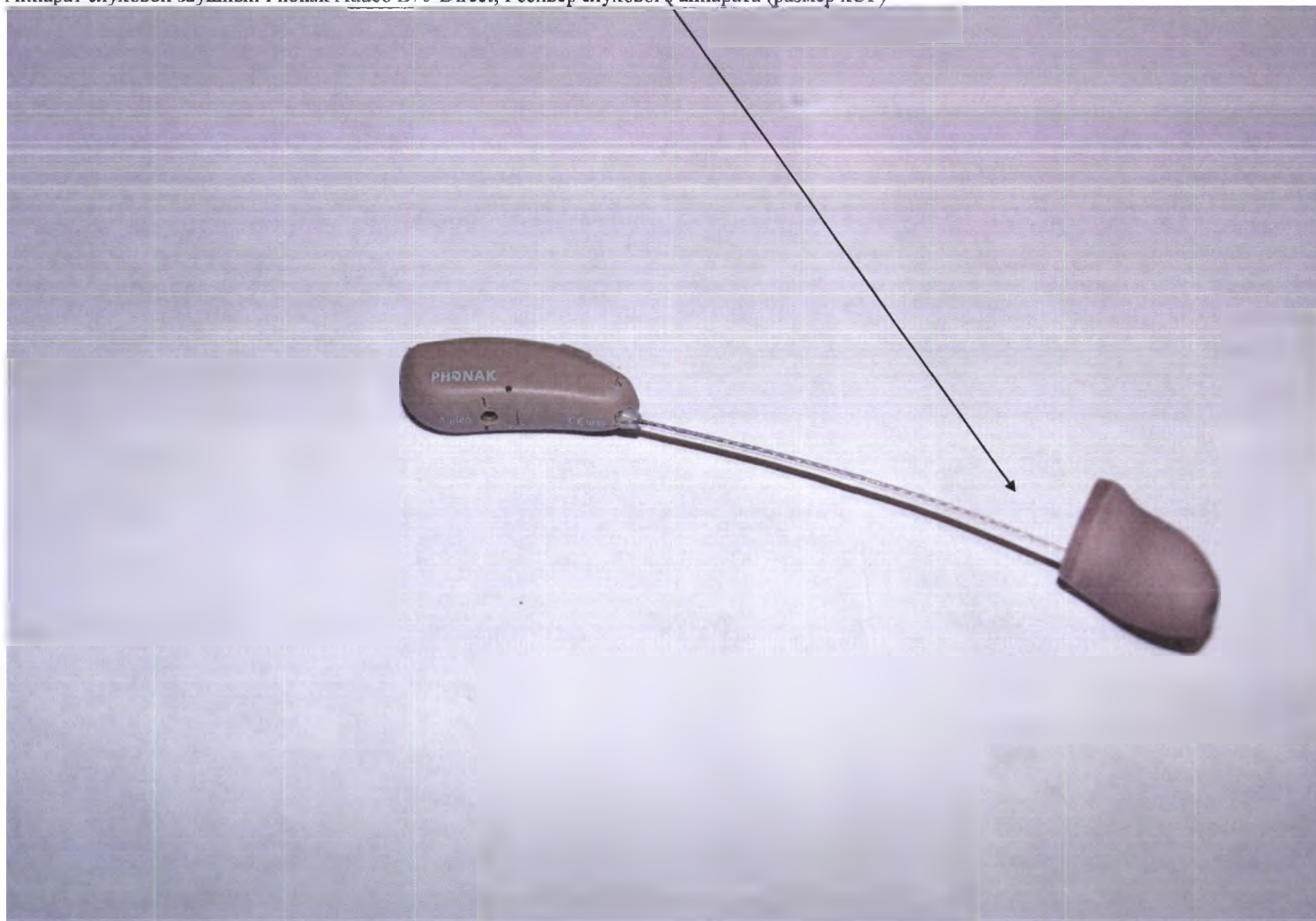
Аппарат слуховой заушный Phonak Audeo B70-Direct; Ресивер слухового аппарата (размер xUP)
