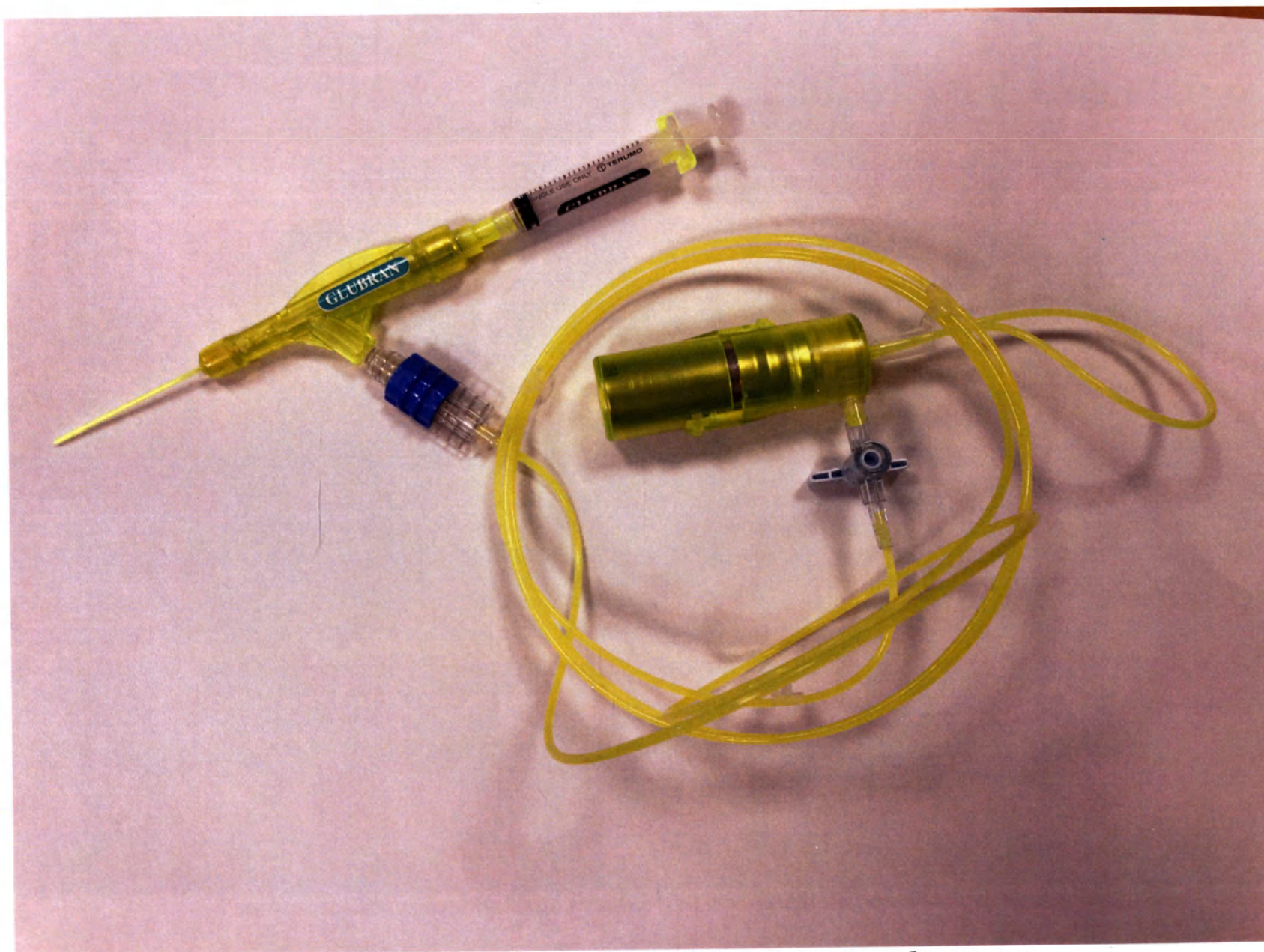
Распылитель для хирургического клея G2-NBT-SM-SHORT в собранном виде
