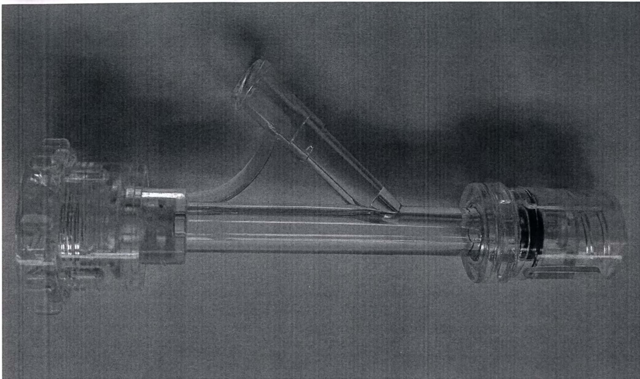
Фото 4. Y-коннектор с гемостатическим клапаном в наборах (исполнение - Y-коннектор с гемостатическим клапаном в наборах тип А 2.0 без удлинителя) Y-коннектор с гемостатическим клапаном в наборах тип А 2.0 без удлинителя
