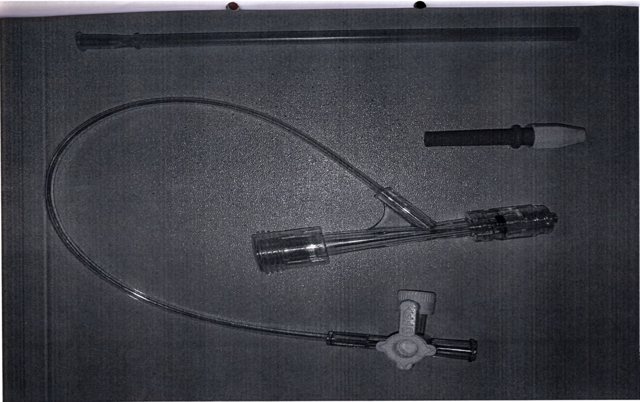
Фото 9. Y-коннектор с гемостатическим клапаном в наборах (исполнение - Y-коннектор с гемостатическим клапаном в наборах тип В 2.0 с удлинителем) Набор
