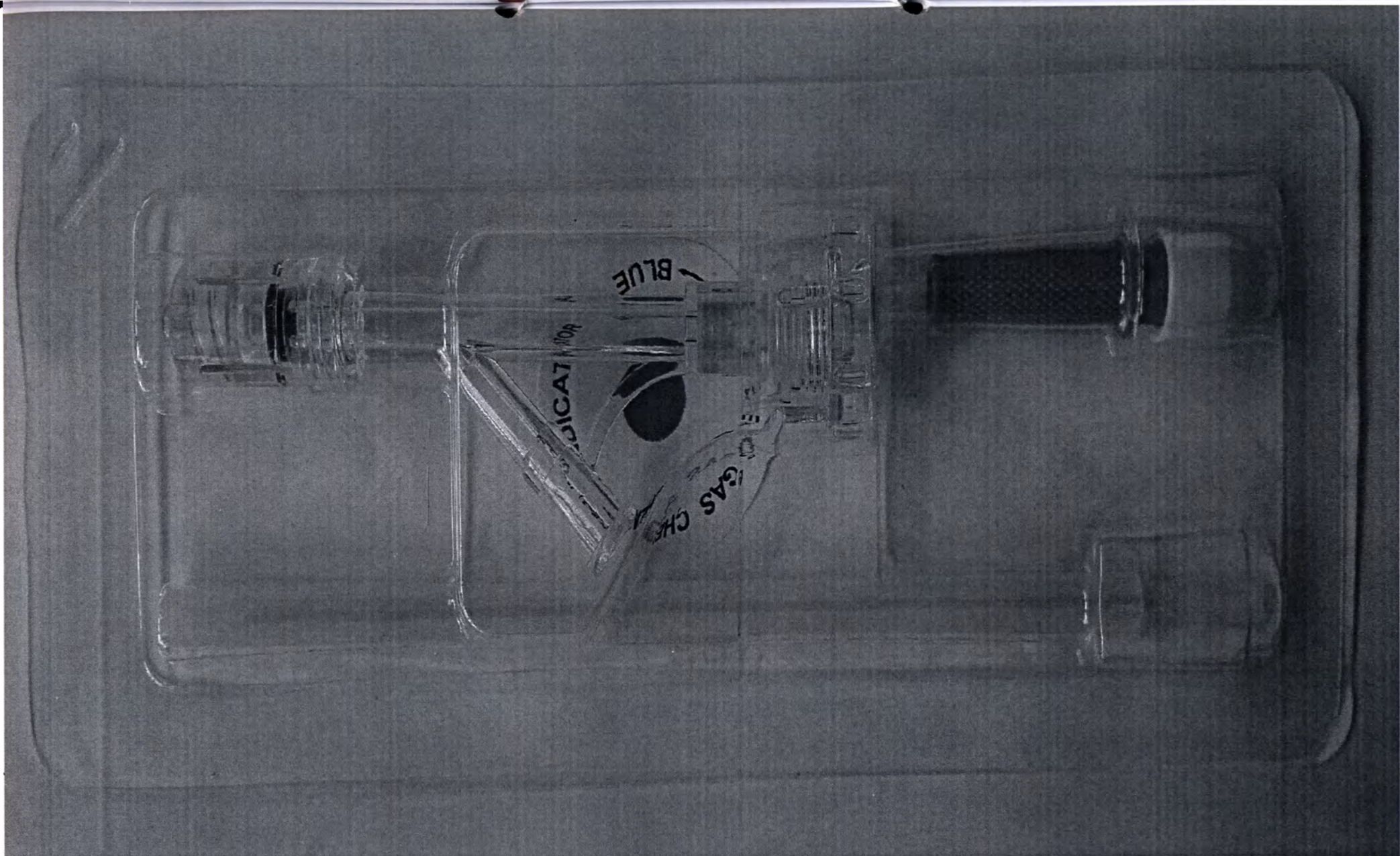
Фото 2. Y-коннектор с гемостатическим клапаном в наборах (исполнение - Y-коннектор с гемостатическим клапаном в наборах тип А 2.0 без удлинителя) в индивидуальной (стерилизационной) упаковке – обратная сторона
