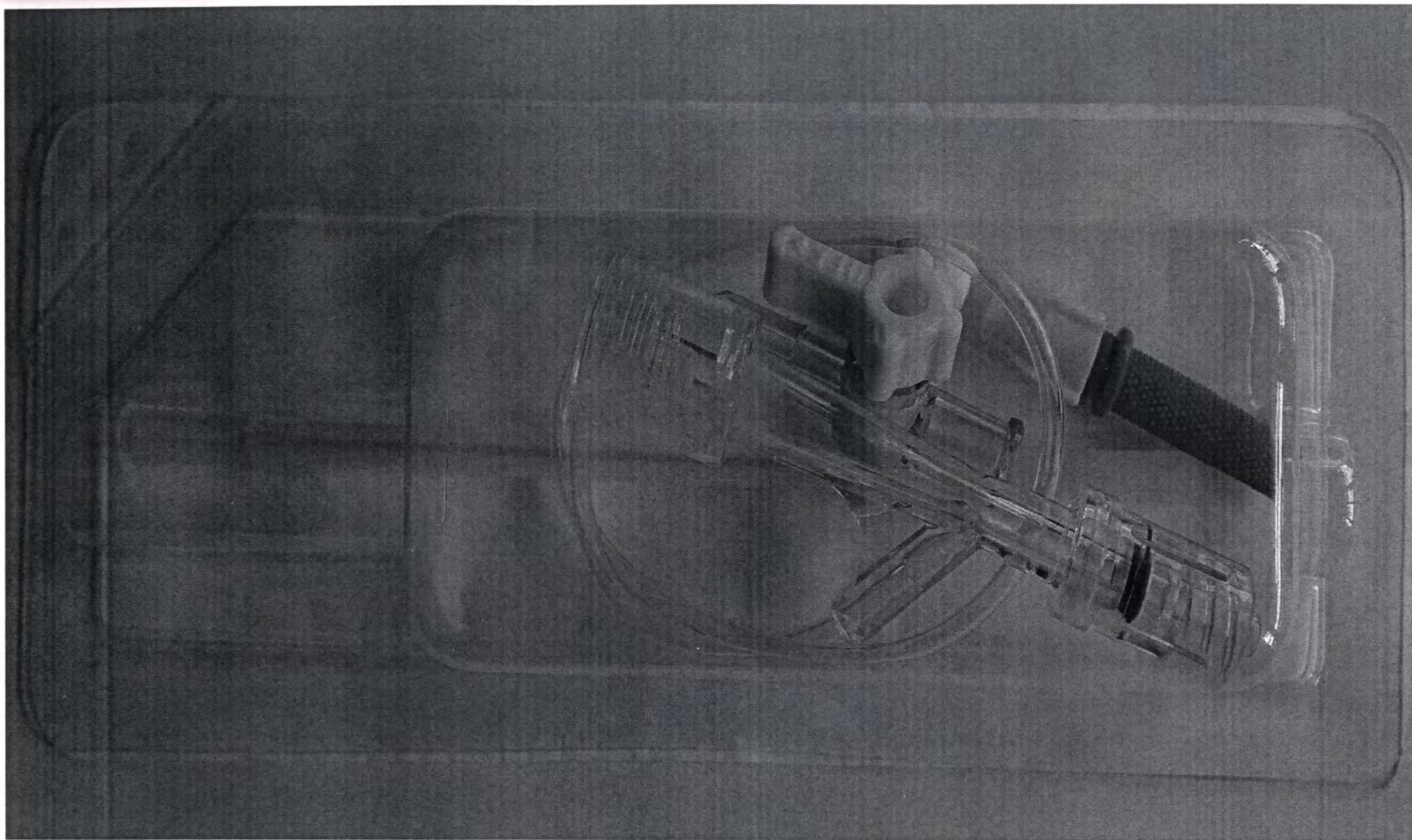
Фото 8. Y-коннектор с гемостатическим клапаном в наборах (исполнение - Y-коннектор с гемостатическим клапаном в наборах тип В 2.0 с удлинителем) в индивидуальной (стерилизационной) упаковке – обратная сторона
