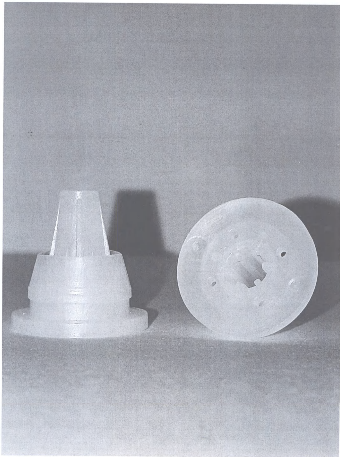
Общий вид пробки капельницы 4111; 4211; 4311; 4411.
