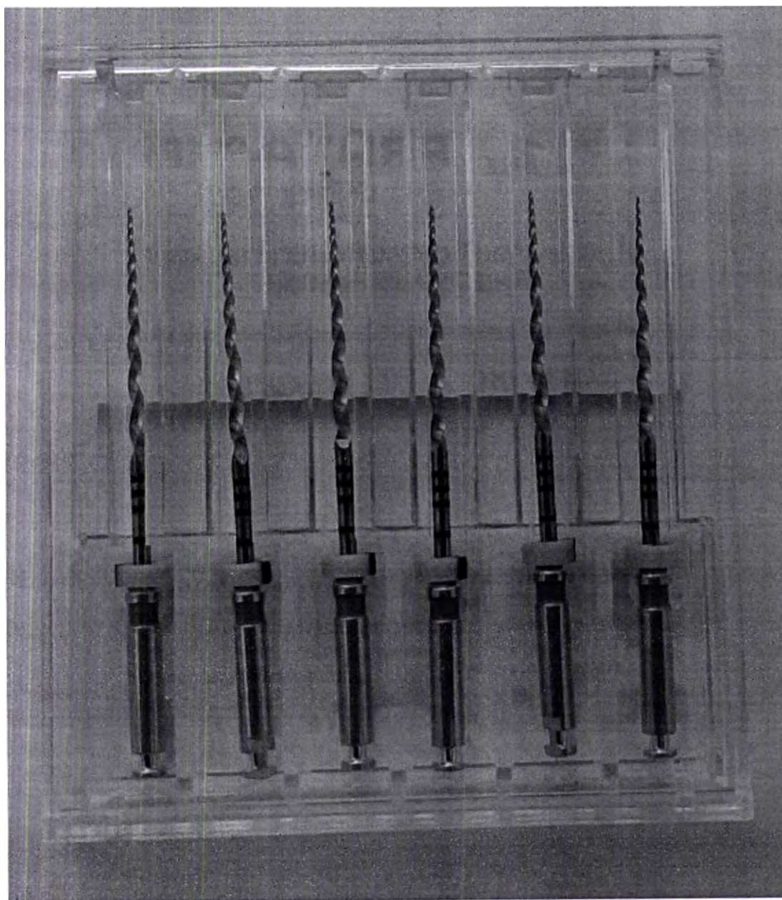
Рис. 75 Инструмент стоматологический эндодонтический Eurofile Ultratapers Engine Use, размер S2, длина 31 мм, никель-титан, 6 шт. в упаковке
