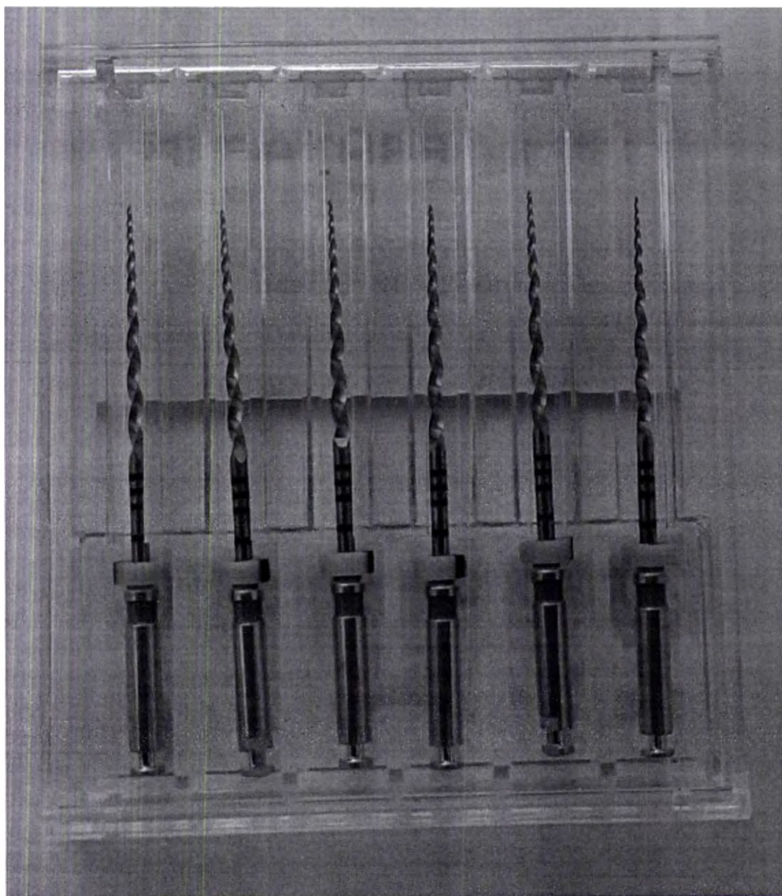
Рис. 77 Инструмент стоматологический эндодонтический Eurofile Ultratapers Engine Use, размер F1, длина 31 мм, никель-титан, 6 шт. в упаковке
