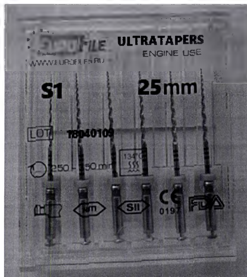
Рис. 60 Маркировка упаковки “Инструмент стоматологический эндодонтический Eurofile Ultratapers Engine Use, размер S1, длина 25 мм, никель-титан, 6 шт. в упаковке”
