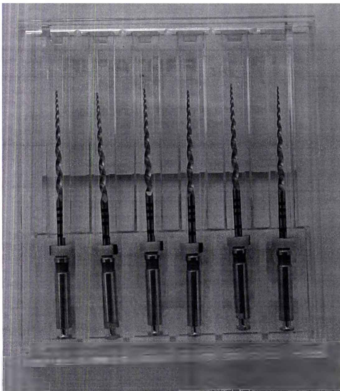
Рис. 81 Инструмент стоматологический эндодонтический Eurofile Ultratapers Engine Use, размер F3, длина 31 мм, никель-титан, 6 шт. в упаковке
