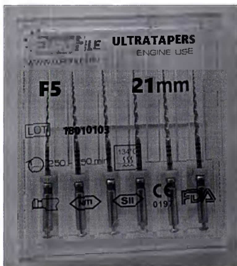
Рис. 58 Маркировка упаковки "Инструмент стоматологический эндодонтический Eurofile Ultratapers Engine Use, размер F5, длина 21 мм, никель-титан, 6 шт. в упаковке"
