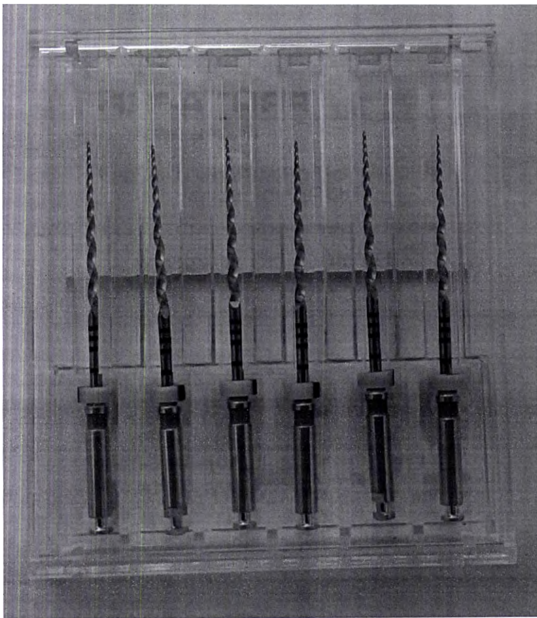
Рис. 73 Инструмент стоматологический эндодонтический Eurofile Ultratapers Engine Use, размер S1, длина 31 мм, никель-титан, 6 шт. в упаковке
