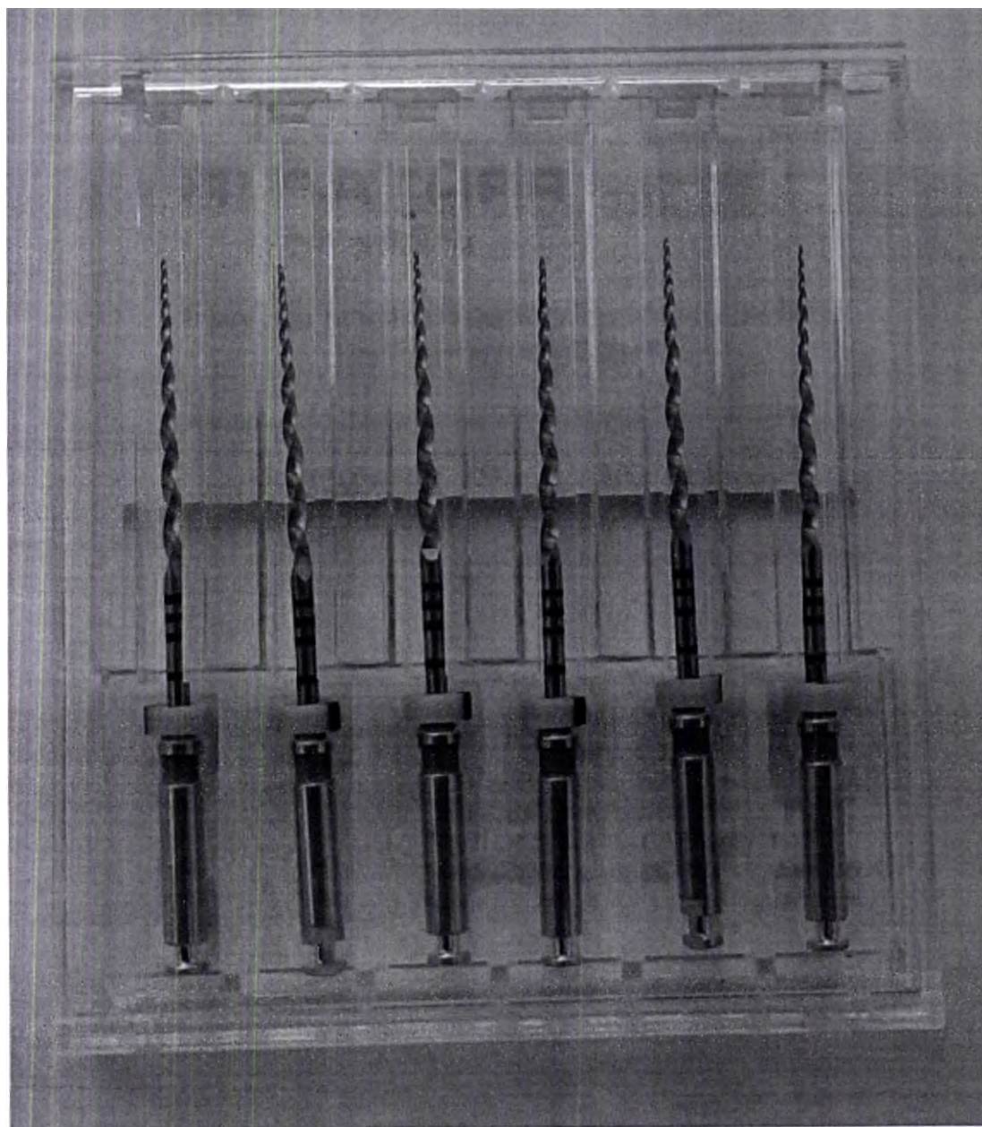
Рис. 91 Инструмент стоматологический эндодонтический Eurofile Ultratapers Engine Use, размер D2, длина 18 мм, никель-титан, 6 шт. в упаковке
