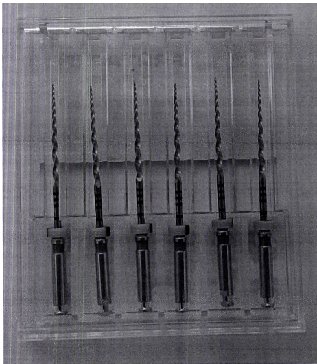
Рис. 59 Инструмент стоматологический эндодонтический Eurofile Ultratapers Engine Use, размер S1, длина 25 мм, никель-титан, 6 шт. в упаковке
