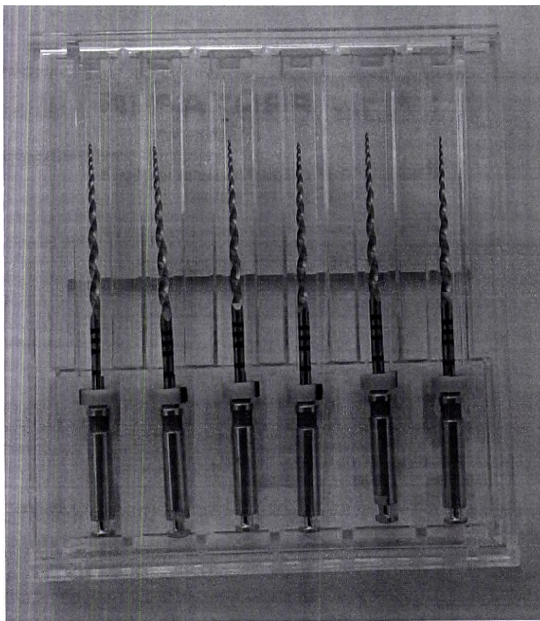
Рис. 61 Инструмент стоматологический эндодонтический Eurofile Ultratapers Engine Use, размер S2, длина 25 мм, никель-титан, 6 шт. в упаковке
