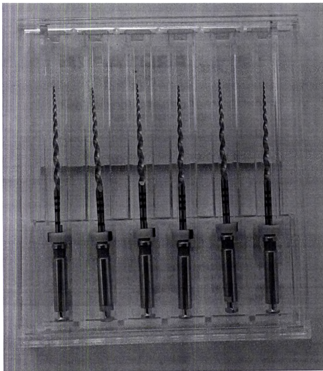
Рис. 83 Инструмент стоматологический эндодонтический Eurofile Ultratapers Engine Use, размер F4, длина 31 мм, никель-титан, 6 шт. в упаковке
