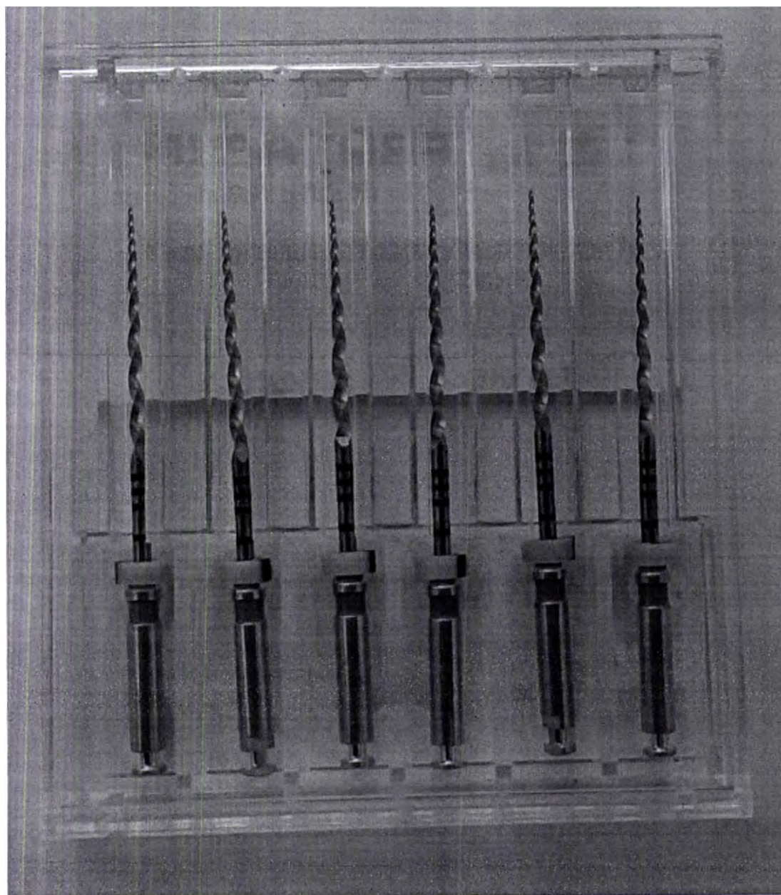
Рис. 85 Инструмент стоматологический эндодонтический Eurofile Ultratapers Engine Use, размер F5, длина 31 мм, никель-титан, 6 шт. в упаковке
