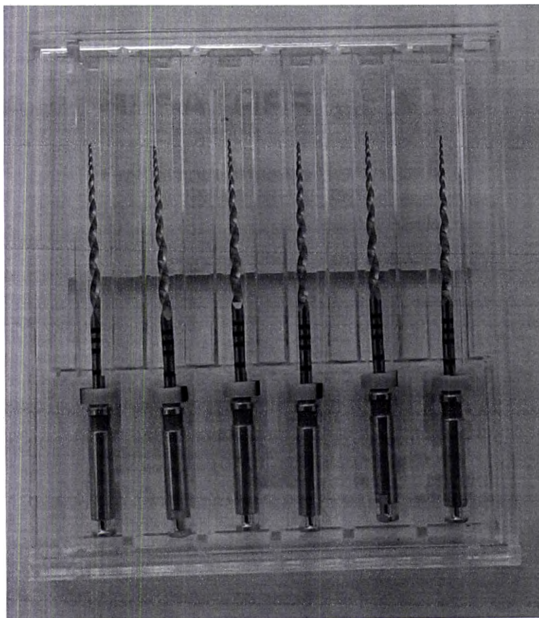
Рис. 51 Инструмент стоматологический эндодонтический Eurofile Ultratapers Engine Use, размер F2, длина 21 мм, никель-титан, 6 шт. в упаковке
