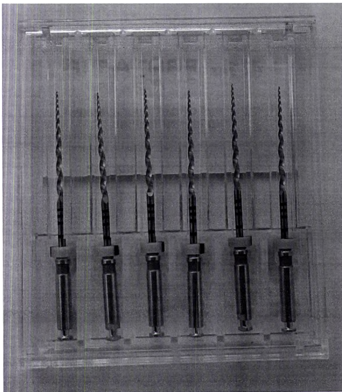
Рис. 45 Инструмент стоматологический эндодонтический Eurofile Ultratapers Engine Use, размер S1, длина 21 мм, никель-титан, 6 шт. в упаковке
