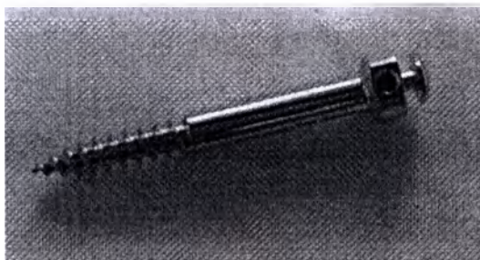
Фото 5 Минивинты серии А-1PIZC с половинной нарезкой и круглым отверстием диаметром 2,0 мм, длина 17 мм, REF A-1PIZC -212017
