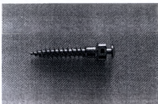
Фото 3 A-1PS с прямоугольным отверстием (модель с торком) диаметром 2,0 мм, длина 12 мм, REF A-1PS-222012
