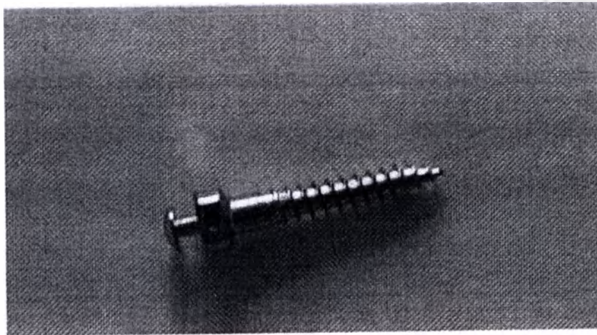
Фото 7 Минивинты серии A-1P с половинной нарезкой и круглым отверстием диаметром 1,5 мм, длина 8 мм, REF A-1P -211508
