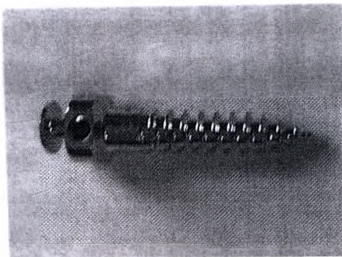
Фото 9 Минивинты серии 1,4 V с круглым отверстием диаметром 1,4 мм, длина 8 мм, REF A-1P V-201405
