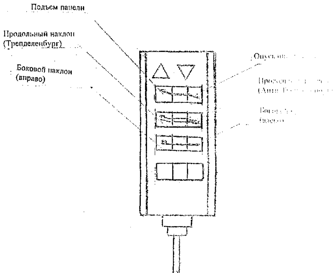
Рис.17 Пульт управления.
