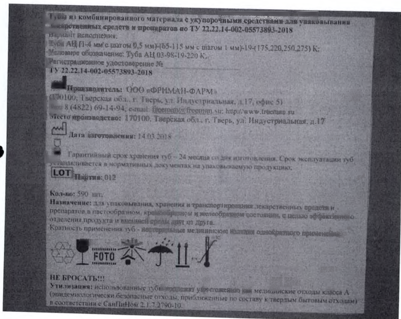
Рисунок 12 – Маркировка корпуса тубы (крупным планом) и этикетка. Туба АЦ (1-4 мм с шагом 0,5 мм)- (65-115 мм с шагом 1 мм)-19-(175,220,250,275) К; Условное обозначение: Туба АЦ 03-98-19-220 К;
