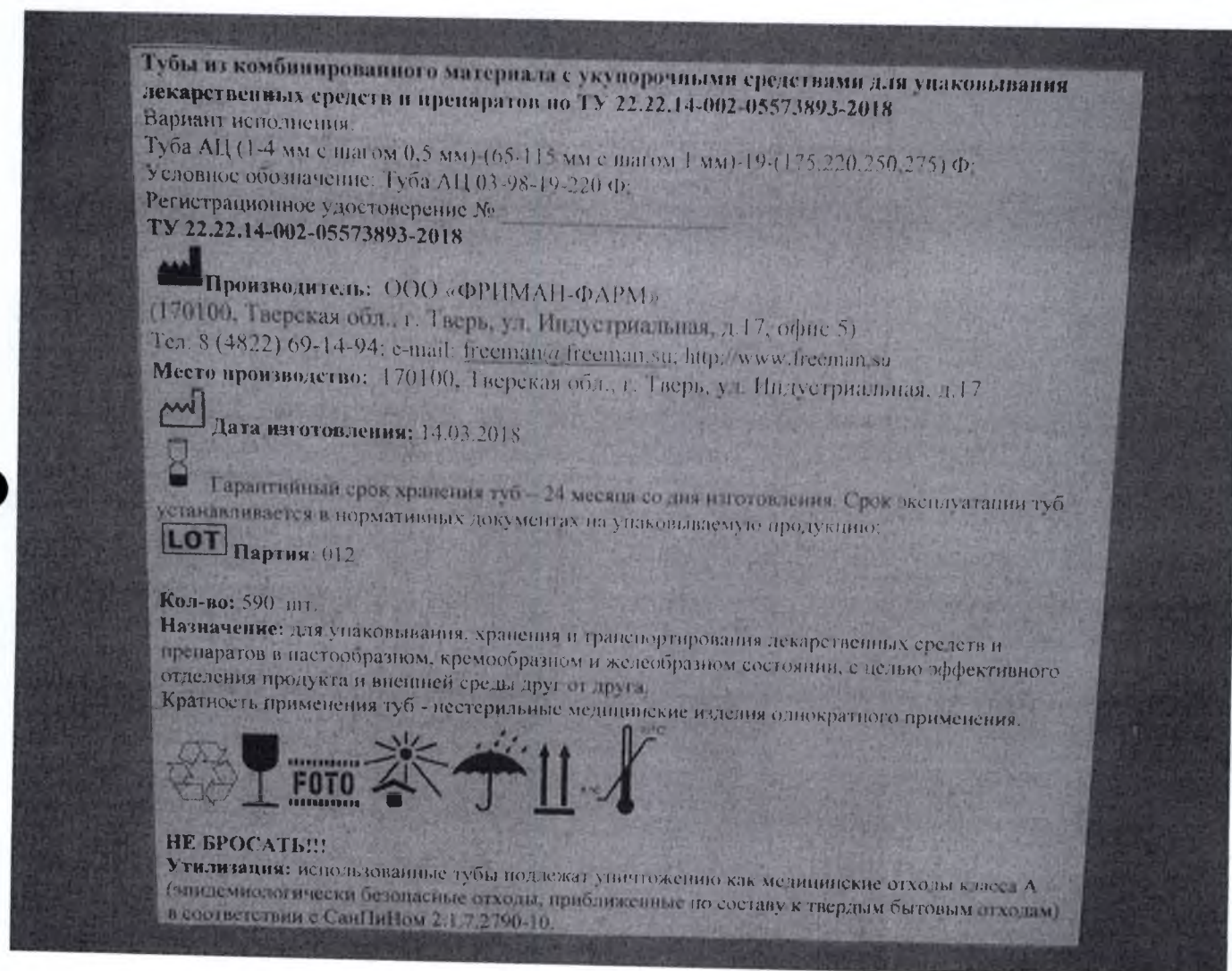
Рисунок 14 – Маркировка корпуса тубы (крупным планом) и этикетка. Туба АЦ (1-4 мм с шагом 0,5 мм)-(65-115 мм с шагом 1 мм)-19-(175,220,250,275) Ф; Условное обозначение: Туба АЦ 03-98-19-220 Ф;
